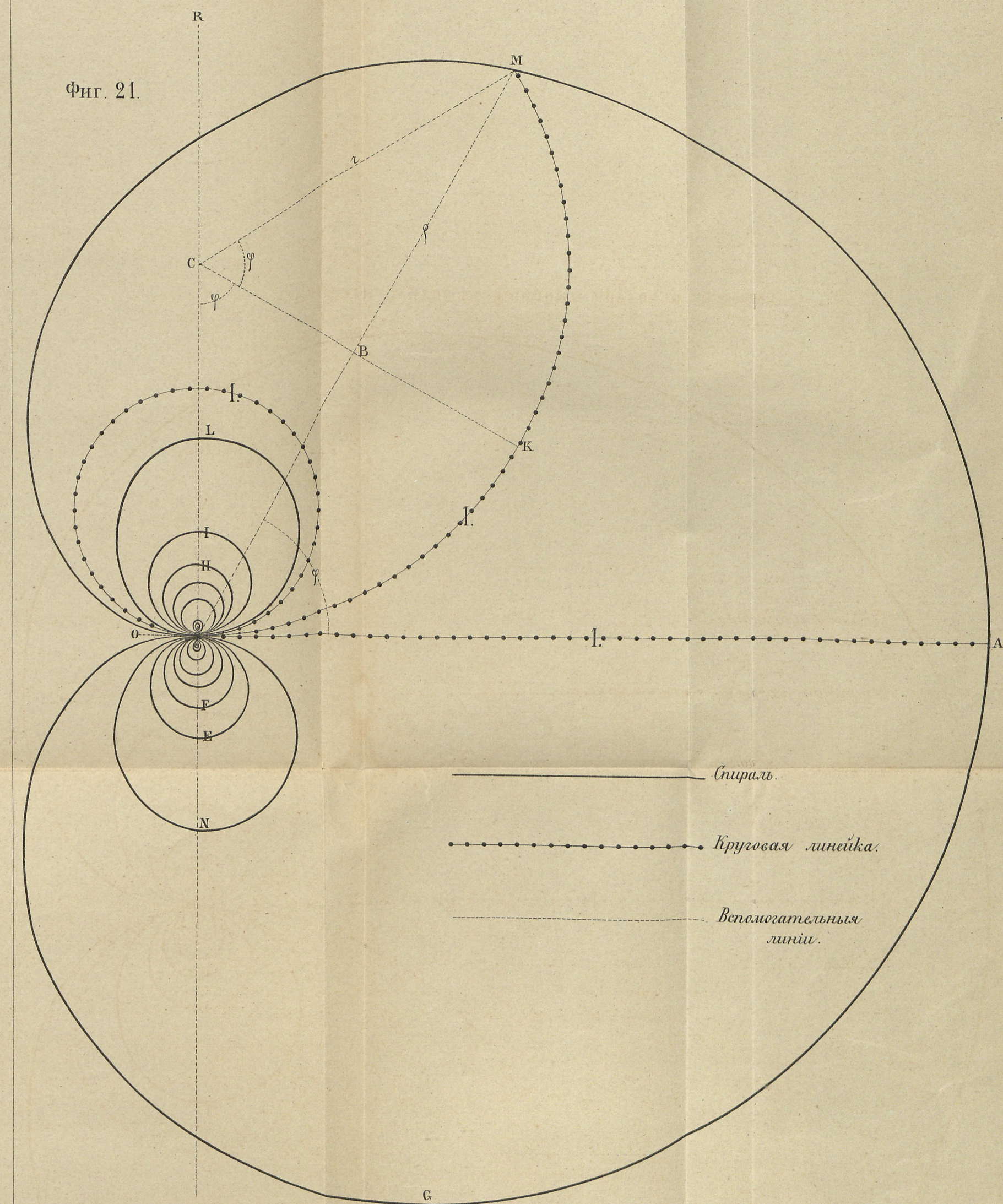
Спираль, чертимая концом круговой линейки.
