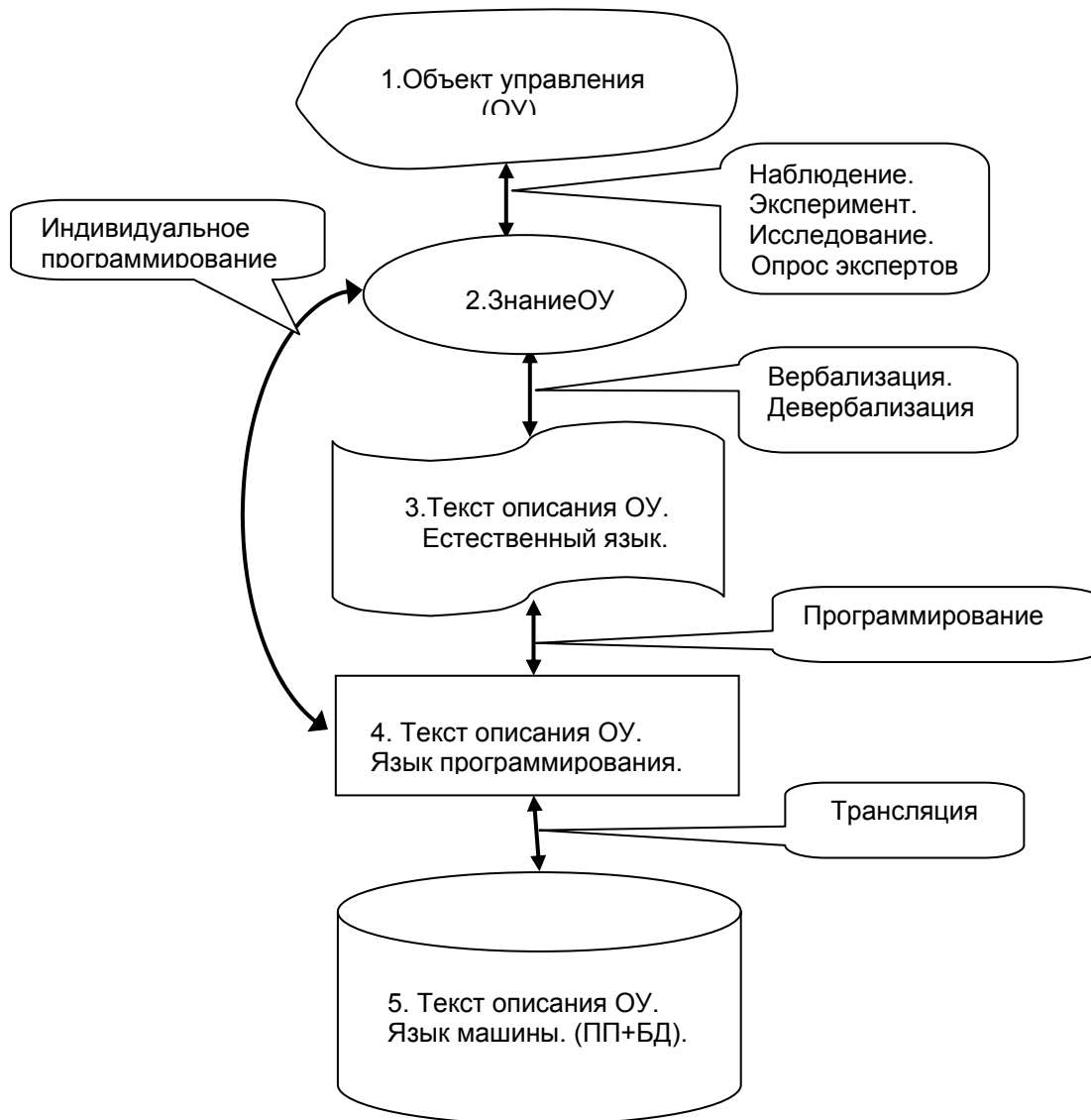
Рис. 4. Построение машинной модели объекта управления.
