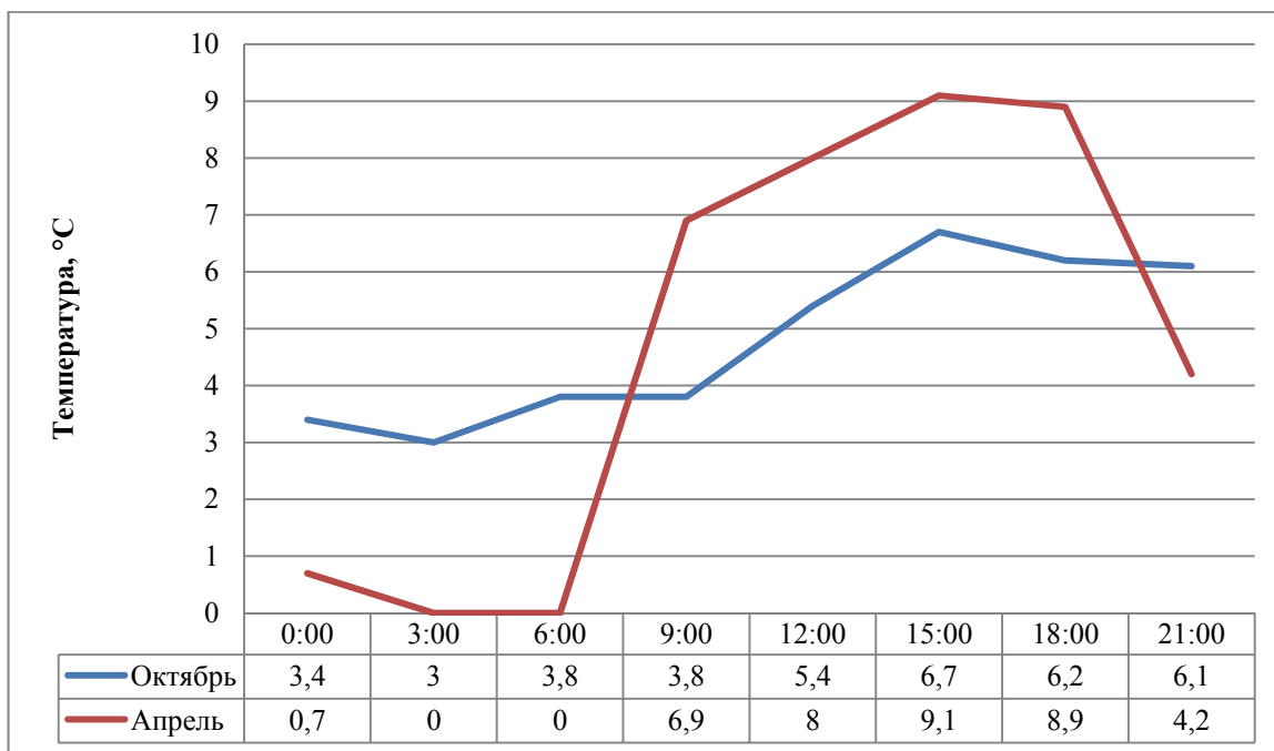
Рисунок 6. Сводная детализация изменения температуры в течение суток (15 октября и 13 апреля) для Москвы
