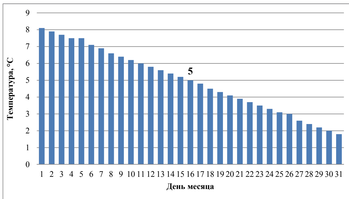
Рисунок 4. Ежесуточные нормы средней температуры воздуха октября для Москвы
