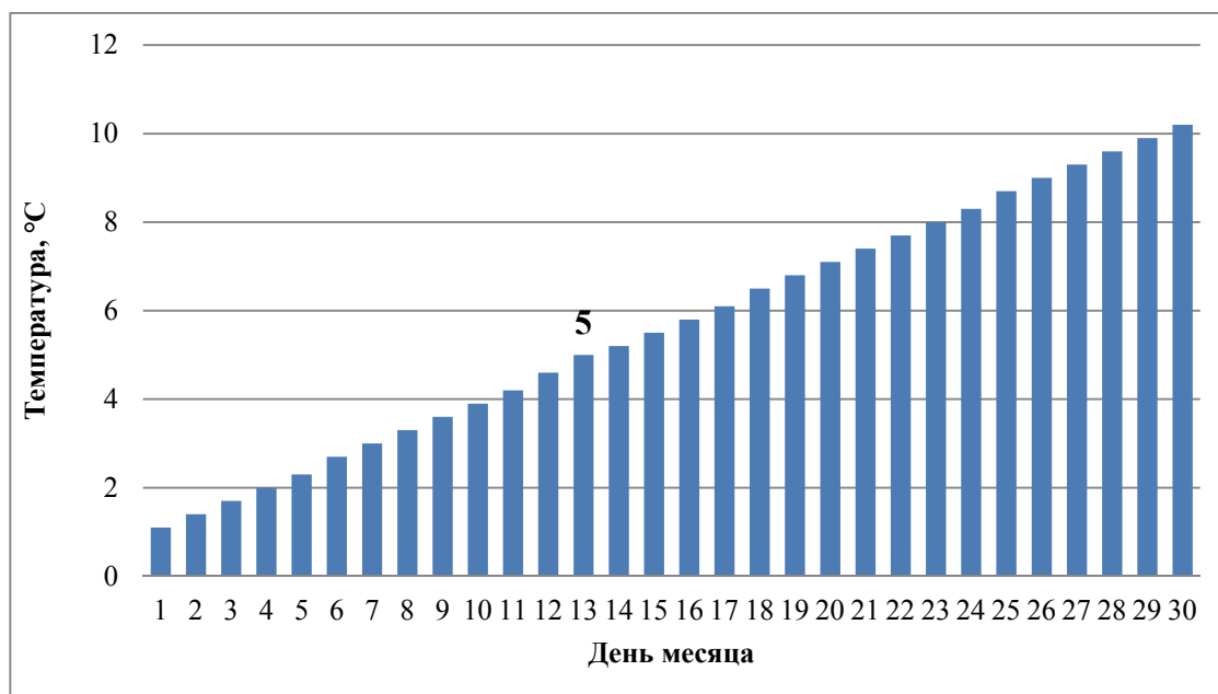
Рисунок 5. Ежесуточные нормы средней температуры воздуха апреля для Москвы
