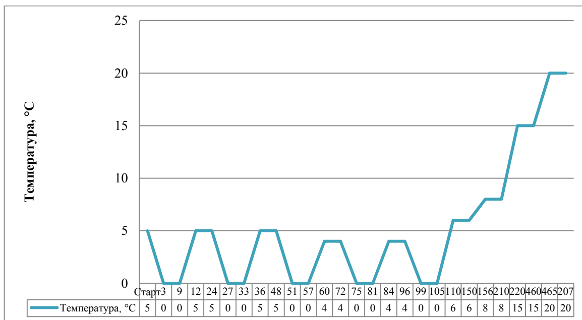
Рисунок 7. Графическая модель климатических испытаний
