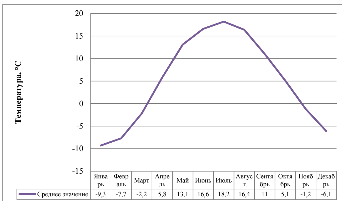
Рисунок 1. Значения среднесуточной температуры для Москвы
