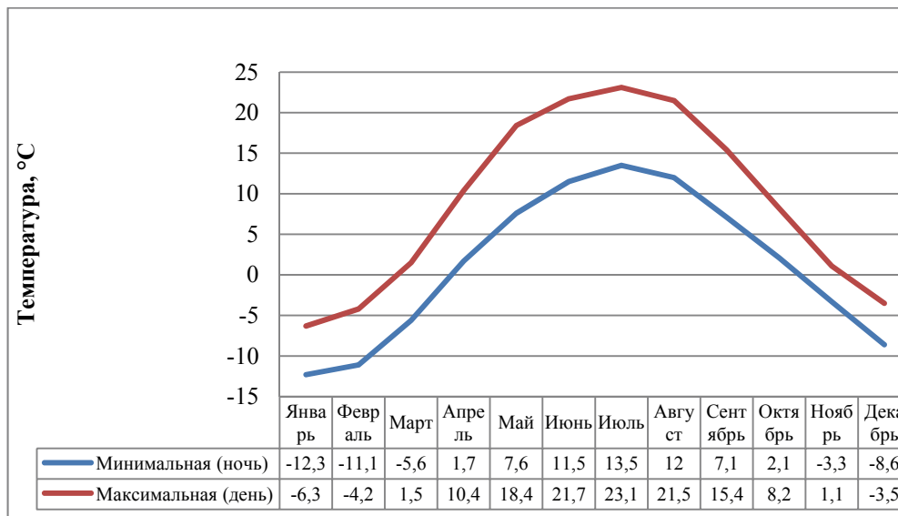
Рисунок 2. Суточные колебания температуры воздуха для Москвы
