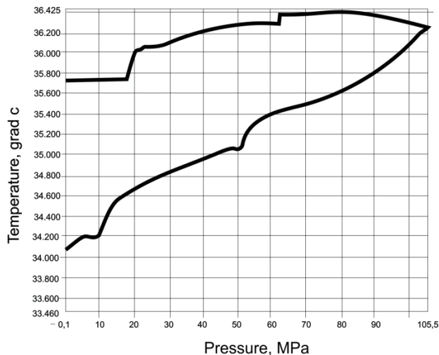
Рисунок 6. Зависимость температуры нонадекана «Ч» C19H40 от давления
