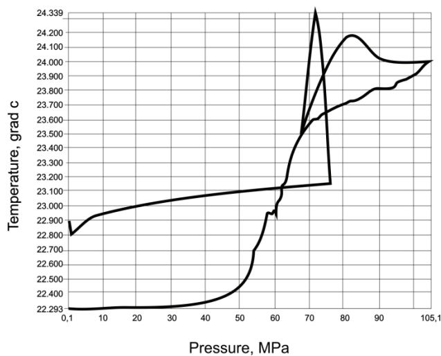
Рисунок 8. Зависимость температуры бензола от давления
