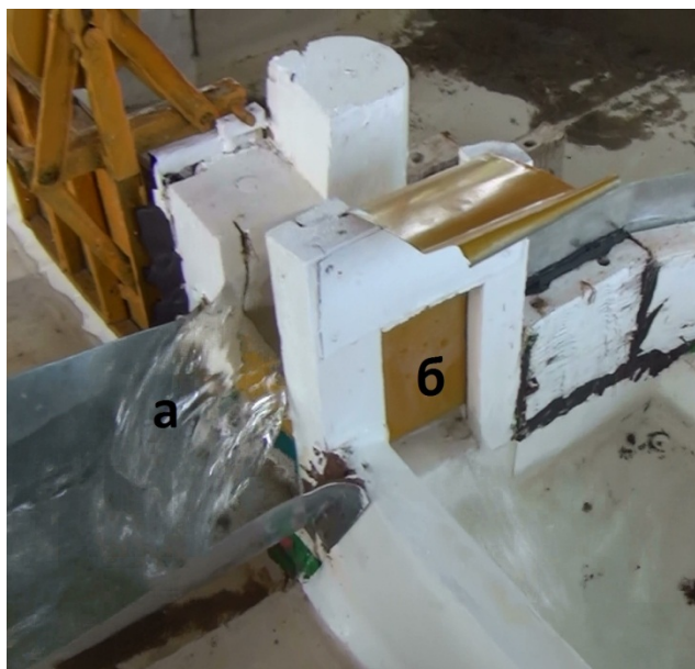
Рисунок 2. Вид струи, переливающейся через сдвоенный затвор промывного тракта, (а) и вид истечения из-под плоского затвора зимнего водозабора (б) на модели
