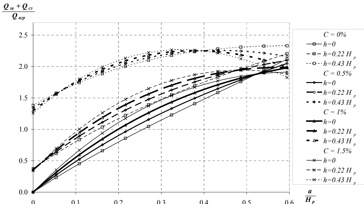
Рисунок 5. Расходные характеристики сдвоенного затвора промывного тракта при различных открытиях затвора зимнего водозабора и концентрациях шуги
