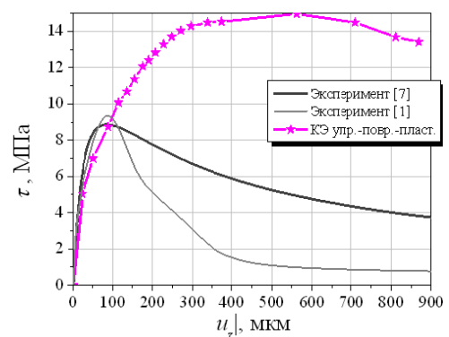
Рисунок 5.5. Зависимость касательного напряжения сцепления от смещения арматуры
