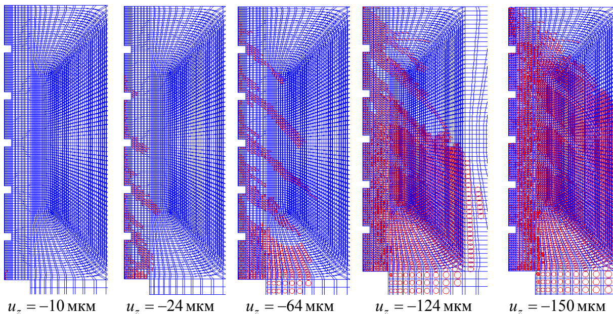
Рисунок 3.1. Эволюция роста микротрещин с увеличением заданного перемещения нижнего торца арматуры
