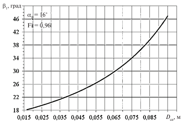
Рис. 8. Зависимость \beta_1(D_{cp})
