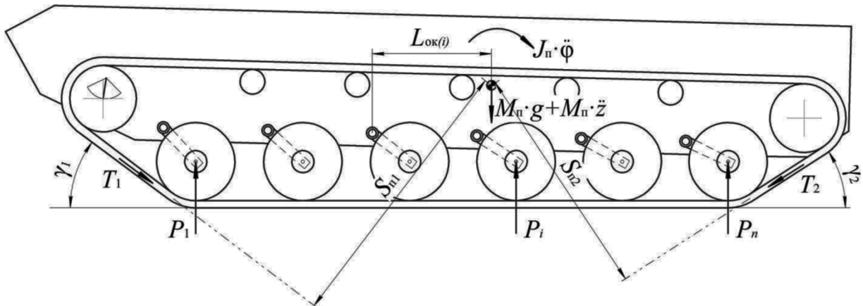
Рис. 4. Расчетная схема сил, действующих на ходовую часть: M_{п} – подрессоренная масса машины; g – ускорение свободного падения; P_i – упругая сила подвески, приведенная к i -му опорному катку; T_1 – сила, действующая в передней ветви обвода; T_2 – сила, действующая в задней ветви обвода, S_{п1} и S_{п2} – плечи моментов сил натяжения гусениц относительно центра подрессоренной массы; n – число опорных катков на борт; J_{п} – момент инерции подрессоренной массы
