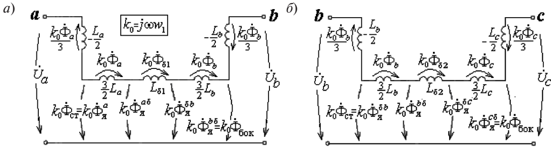
Рис. 2. 4Т-схемы замещения двухобмоточных a, b -трансформатора (а) и b, c -трансформатора (б)
