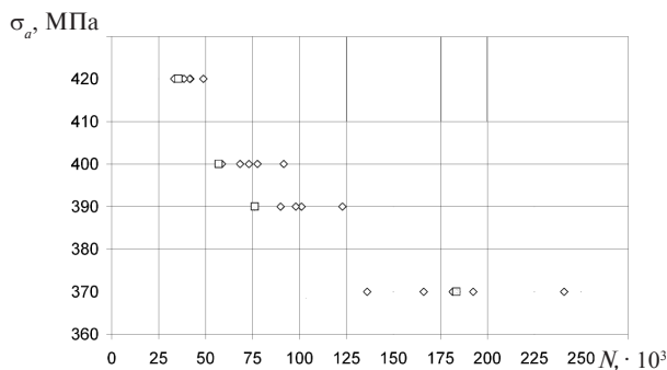
Рис. 7. Сопоставление экспериментальной и вычисленной при моделировании долговечности образцов для пяти распределений типа «б» ( \square — эксперимент; \diamond — моделирование накопления повреждений)
