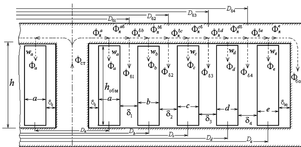
Рис. 1. Магнитные потоки в стали и окне пятиобмоточного бронеового трансформатора
