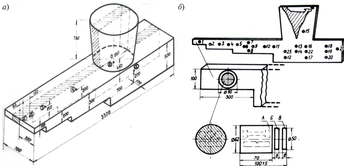
Рис. 1. Общий вид отливки «Проба ступенчатая» (а) с указанием мест расположения термпар (1–6) и осевого продольного темплета (заштриховано), а также расположение контрольных участков (1–22) для оценки качества литого металла и вырезки образцов для механических испытаний (б)
