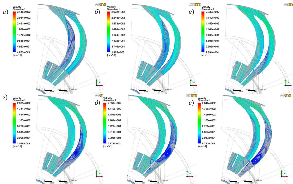
Рис. 6. Линии тока в обратно направляющем аппарате на средней по высоте лопасти поверхности тока при различных значениях условного коэффициента расхода (лопатки РК заострены по передней поверхности до средней линии, модель с лабиринтными уплотнениями): а) \Phi = 0,0468 ; б) \Phi = 0,0423 ; в) \Phi = 0,0377 ; г) \Phi = 0,032 ; д) \Phi = 0,0283 ; е) \Phi = 0,0202
