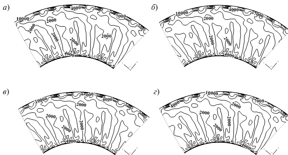
Рис. 3. Изобары избыточного давления торможения (Па) за ступенью при различном взаимном положении лопаток РК и НА: а) начальное положение; б) сдвиг на 2^\circ ; в) сдвиг на 4^\circ ; г) сдвиг на 6^\circ
