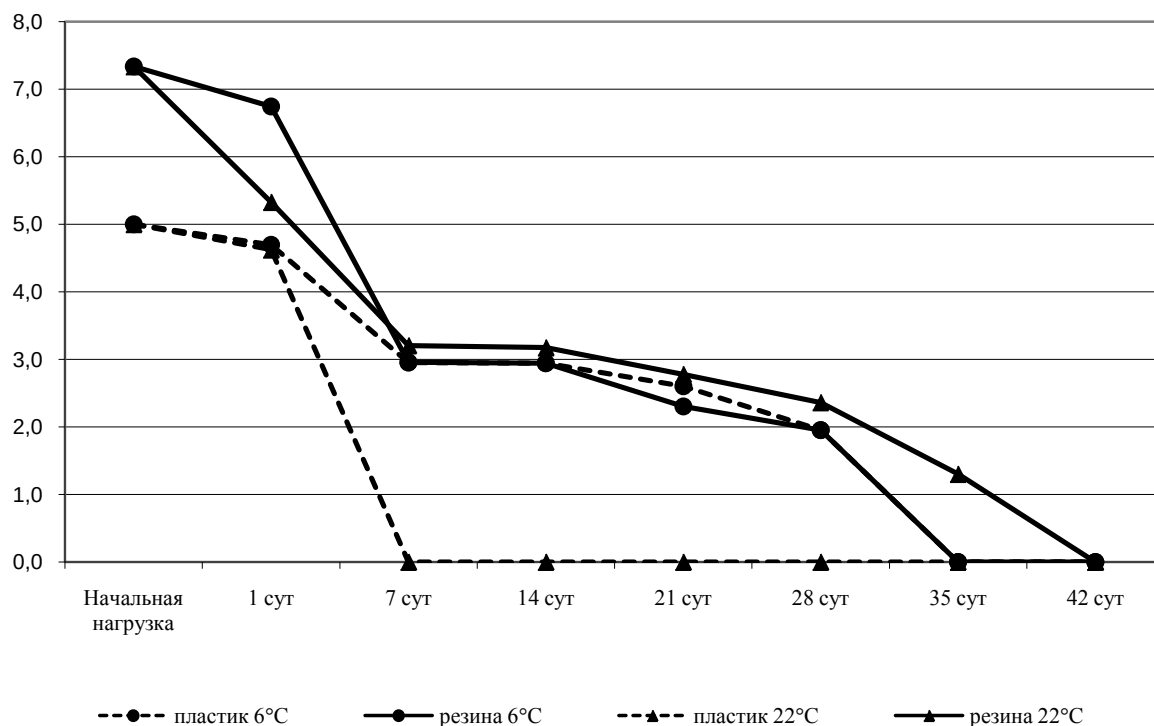
Рис. 1. Выживаемость Pseudomonas aeruginosa , штамм 29
