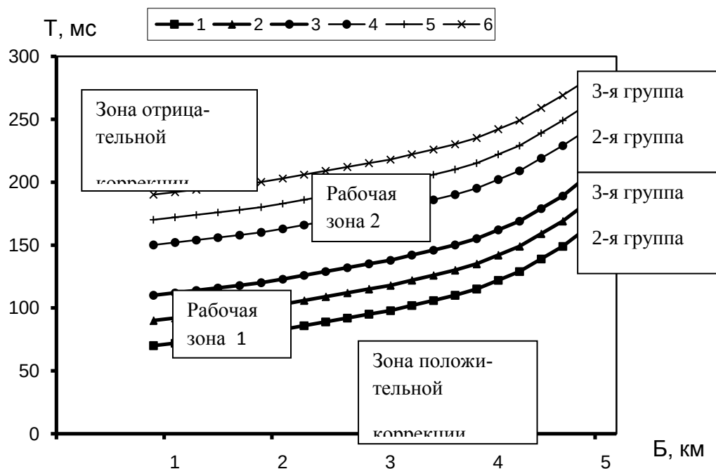
Рис. 1 Рабочие и коррекционные зоны беговых упражнений в зависимости от изменения времени включения икроножной мышцы (1) и прямой мышцы бедра (2)
