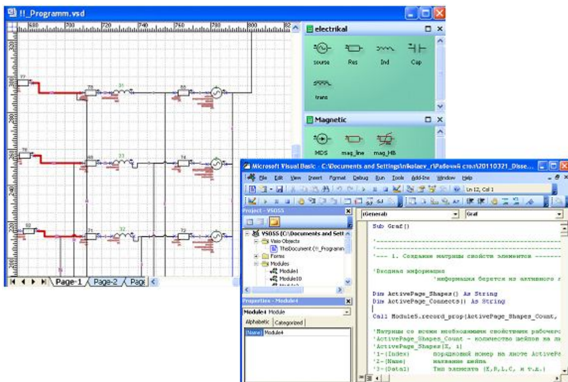
Рис. 6 MS Visio
