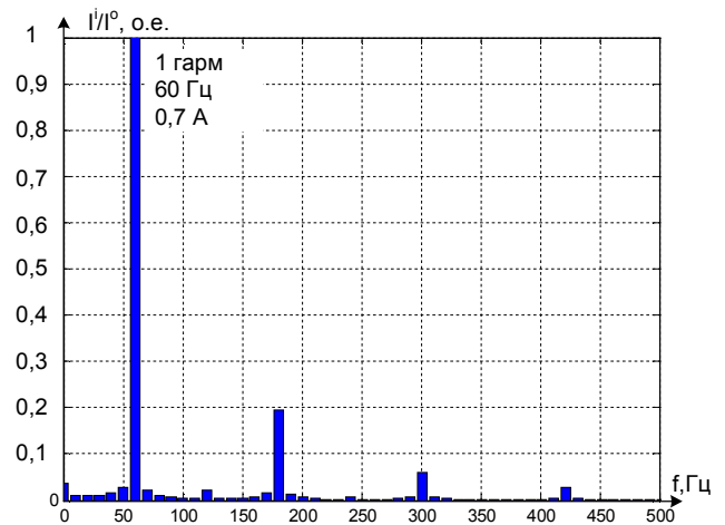
Рис. 5 Гармонический состав тока холостого хода в установившемся режиме работы ( V_n=1,5 Тл)
