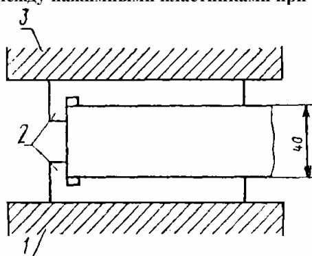
1-нижняя плита пресса; 2 -пластинки; 3 - верхняя плита пресса Черт. 8
