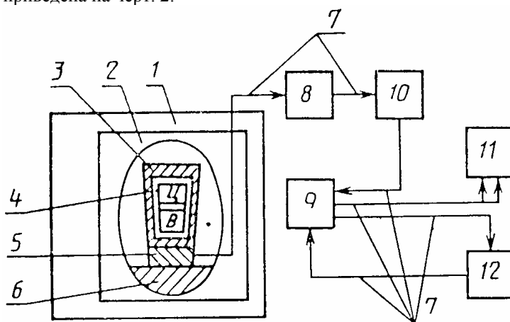
1-термостат; 2 - калориметрический блок; 3 - камера; 4 - ячейка; 5 - тепломер; 6 - теплоотвод; 7 - соединительные кабель; 8 - коммутатор; 9 - калибратор; 10 - предварительный усилитель; 11 - самописец; 12 - интегратор
