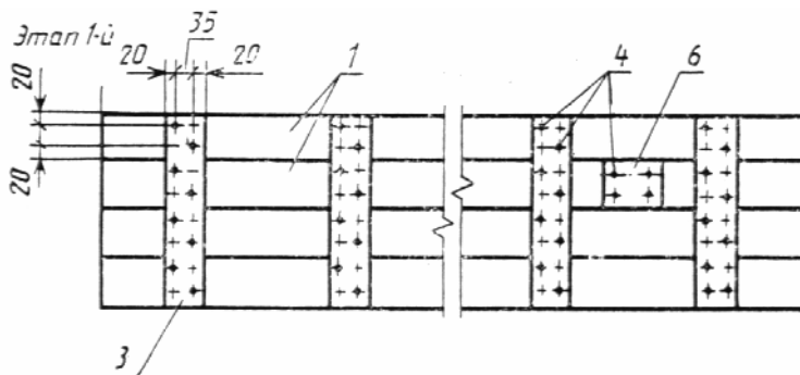
Схема крепления элементов щита
