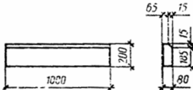
Камни марки БР100.20.8
