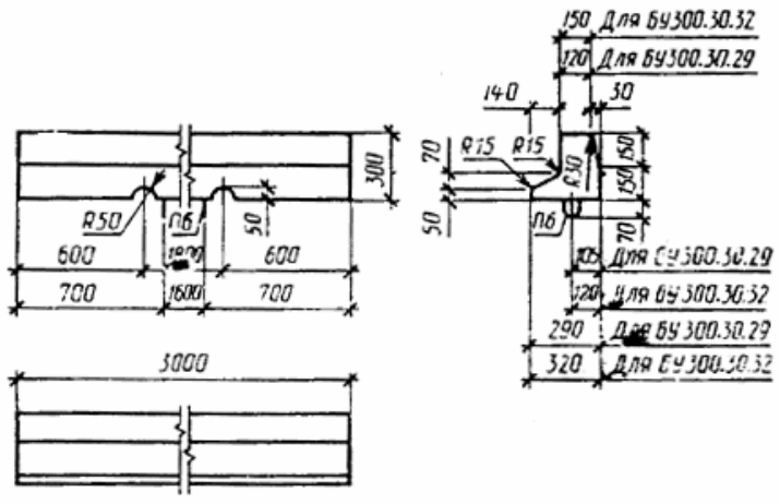
Черт. 6 Камни типа БУП300
