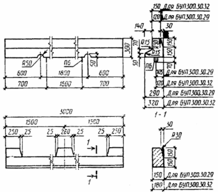
Черт. 7 Камни марки БУП600.30.32-АІV
