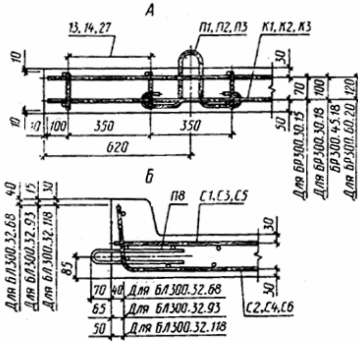
Черт. 18 Арматурные сетки С1 и С2
