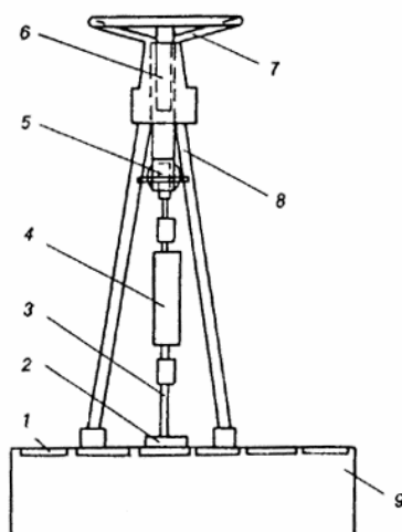
1 — облицовочная плитка; 2 — стальная пластинка; 3 — стержень; 4 — динамометр усилием 5 кН (500 кгс); 5 — шарнир; 6 — винт; 7 — маховое колесо; 8 — тренога; 9 — фрагмент конструкции Черт. 6
