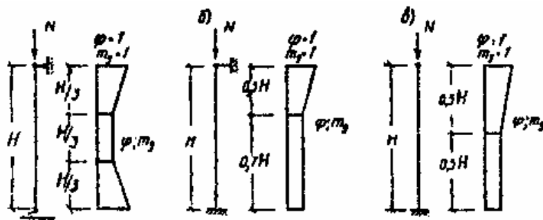
Рис. 4. Коэффициенты \varphi и m_2 по высоте сжатых стен и столбов
