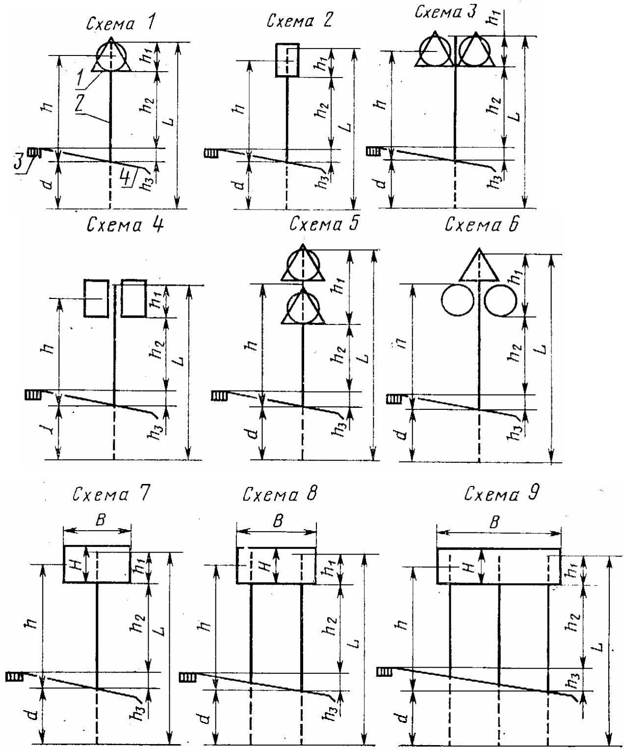
1 - 1 - дорожный знак; 2 - опора; 3 - покрытие автомобильной дороги; 4 - обочина (присыпная берма)
