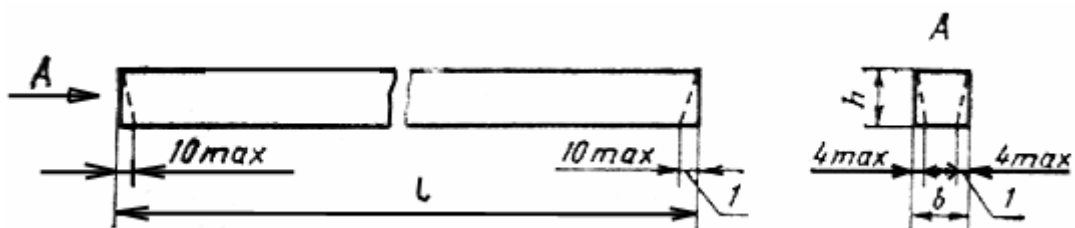
1 - технологический уклон Черт. 1
