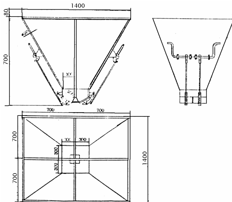
Бункер для камня
