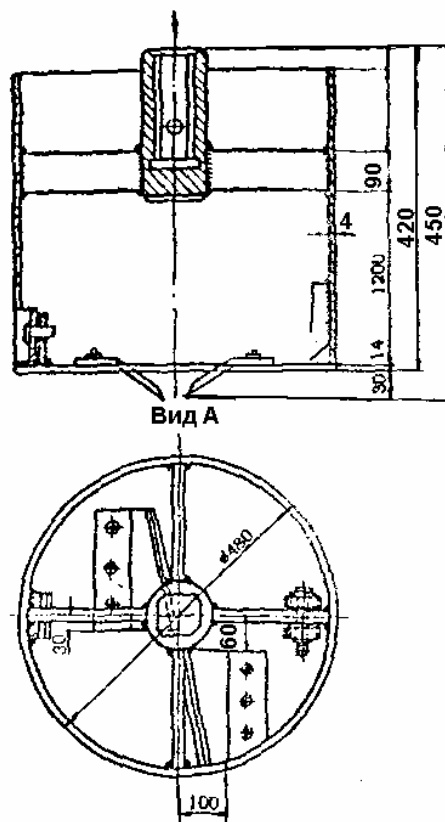
Приспособление для выемки грунта из скважин
