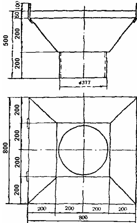
Загрузочная воронка
