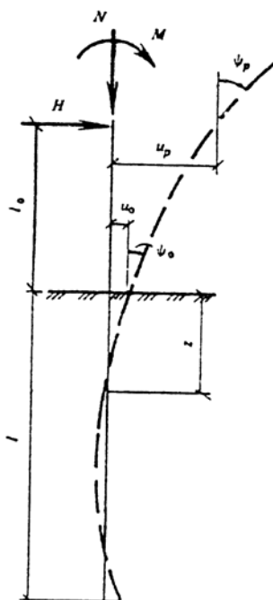
Схема нагрузок на сваю
