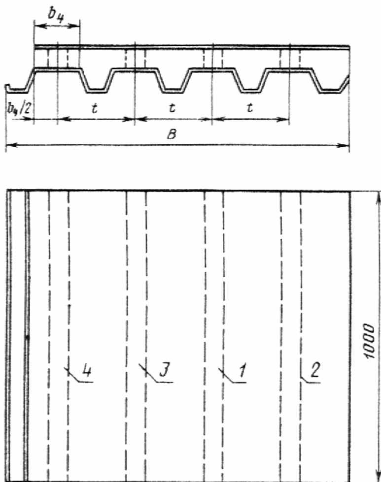
Схема мест вырезки образцов
