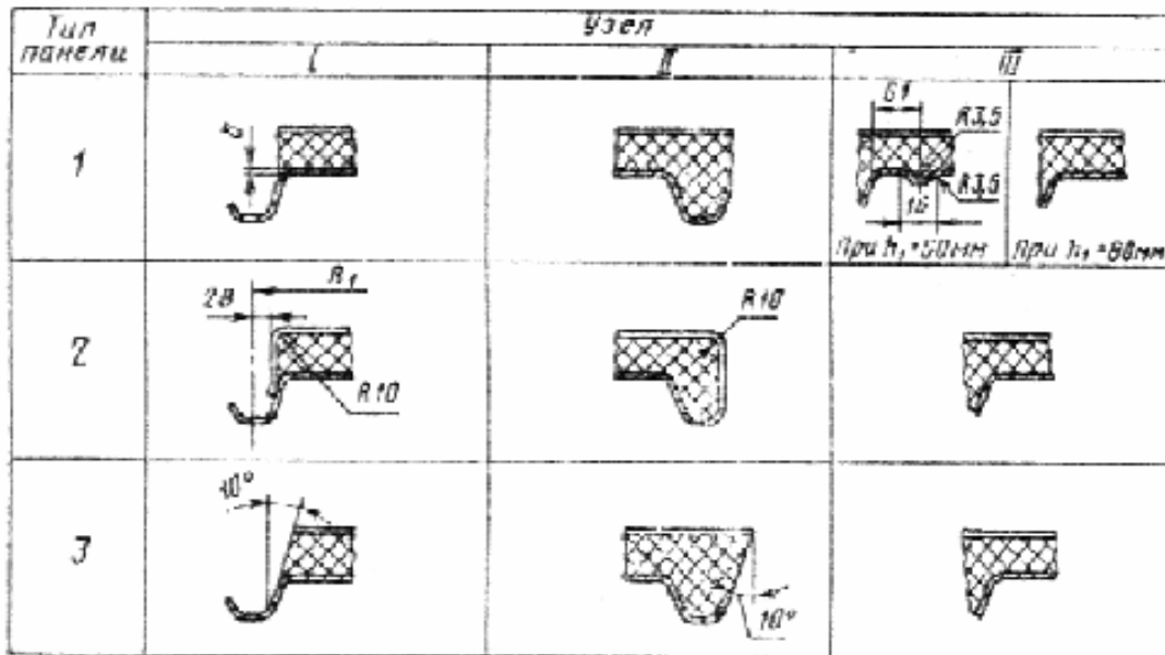
1 - стальной лист; 2 - пенополиуретан; 3 - покровный слой под кровлю Черт.1
