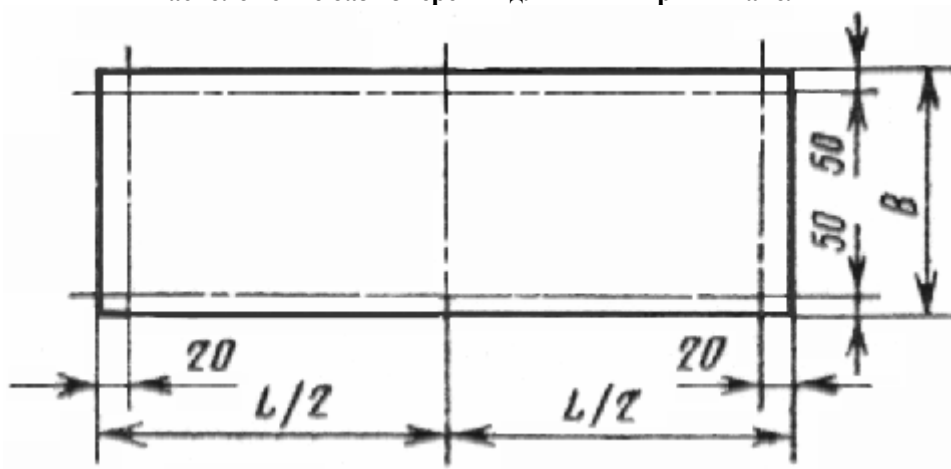
Расположение баз измерения длины и ширины панели
