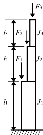
Рис. 25. Схема двухступенчатой колонны
