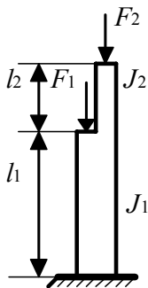
Рис. 24. Схема одноступенчатой колонны
