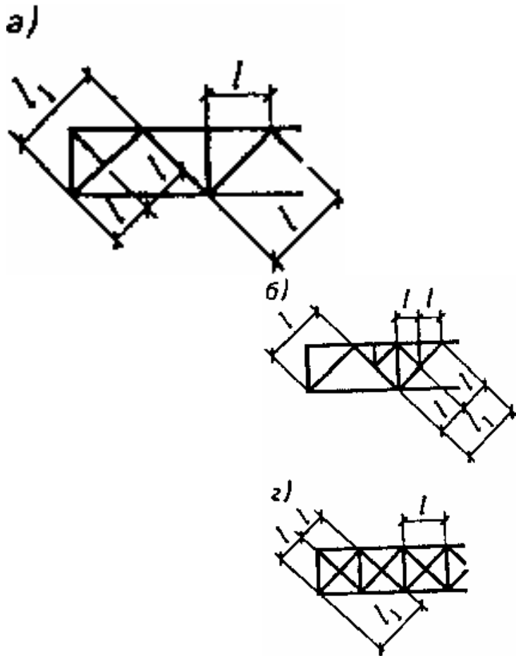
Черт. 6. Схемы решеток ферм для определения расчетной длины элементов
