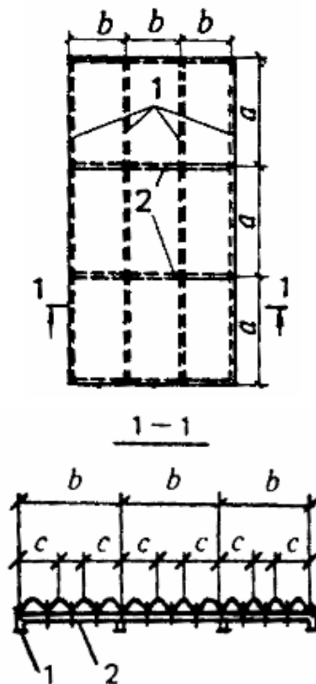
Черт. 14. Схема плиты из гофрированного листа с продольными и поперечными ребрами 1 - продольные ребра; 2- поперечные ребра
