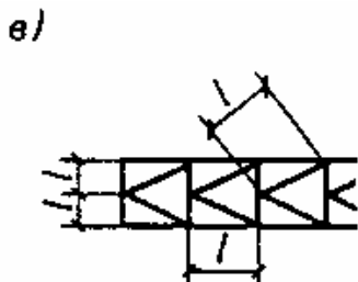
Черт. 6. Схемы решеток ферм для определения расчетной длины элементов
