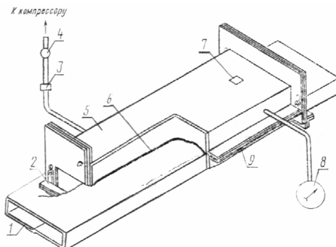
1 — образец; 2 — опора; 3 — трехходовой кран; 4 — вентиль; 5 — короб; 6 — резиновая мембрана; 7 — предохранительный клапан; 8 — манометр; 9 — крепежные уголки
