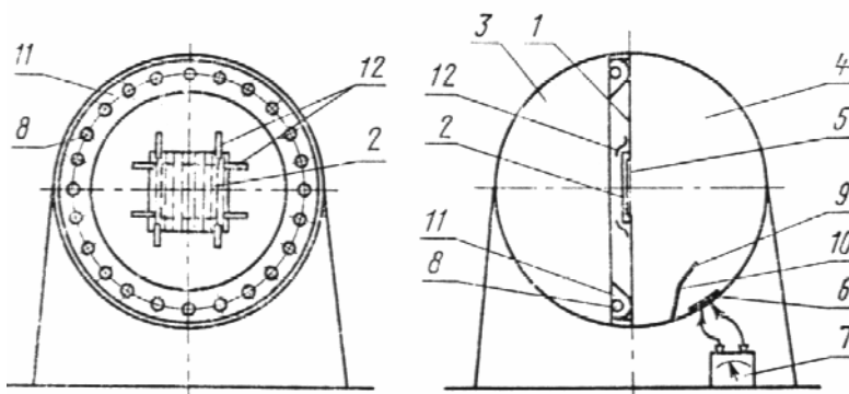
Схема диффузометра
