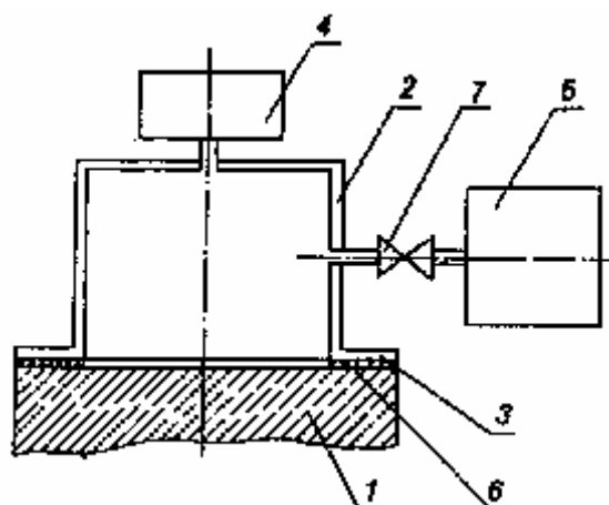
1 — бетонный образец; 2 — камера устройства; 3 — фланец камеры; 4 — вакуумметрический датчик; 5 — вакуум-насос; 6 — герметизирующая мастика; 7 — вентиль
