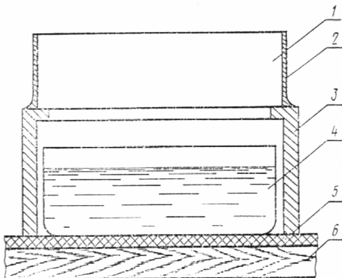
1 — образец ячеистого бетона; 2 — пароизоляция; 3 — металлическая труба; 4 — стеклянная чашка с насыщенным раствором сульфата калия ( K_2SO_4 ); 5 — листовая мягкая резина; 6 — стеллаж
