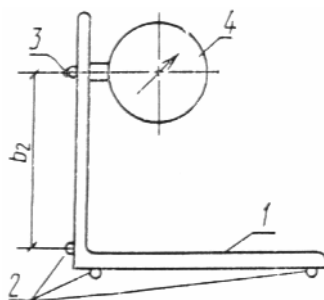
1 — корпус (угольник); 2 — опора; 3 — измерительный стержень индикатора; 4 — индикатор; b_2 — база прибора Черт. 5
