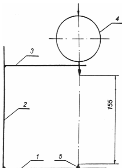
Схема штатива с индикатором часового типа
