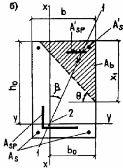
Черт. 7. Форма сжатой зоны в поперечном сечении железобетонного элемента, работающего на косои изгиб
