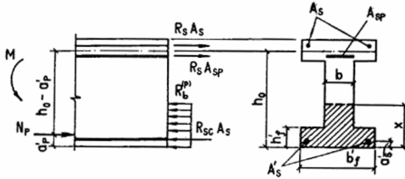
Черт. 30. Схема усилий в поперечном сечении внецентренно обжатого железобетонного элемента полкой в сжатой зоне
