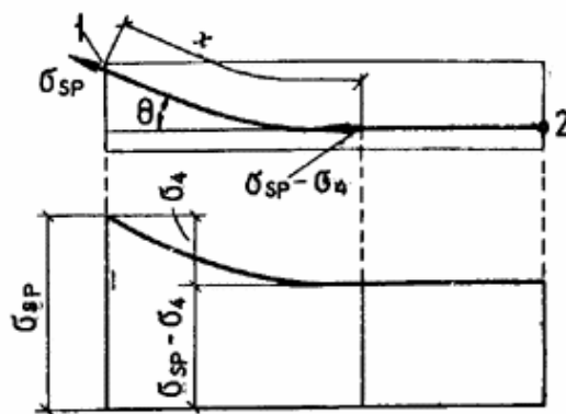
Черт. 1. Схема изменения напряжений в арматуре при наличии трения арматуры о стенки каналов, о поверхность бетона или об обгибающие приспособления
