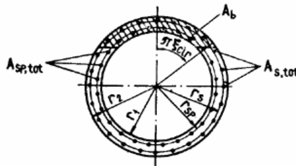
Черт. 28. Схема, принимаемая при расчете кольцевого сечения
