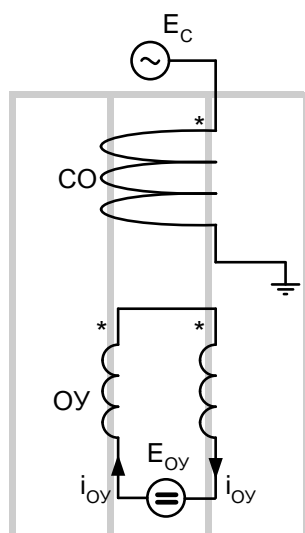
Рисунок 1 - Принципиальная схема магнитного вентиля
