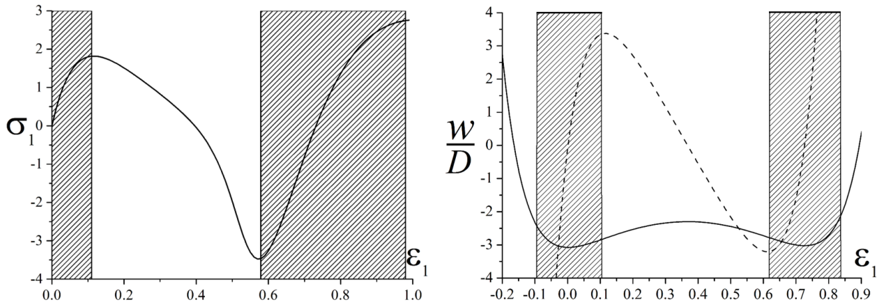
Рис. 3: Слева : одноосное нагружение ( \sigma_2 = 0 ). Справа : профиль потенциальной энергии деформации (сплошная линия) и ее производной по \epsilon_1 (пунктир). Сечение области устойчивости заштриховано.
