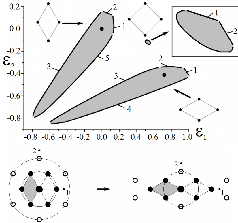
Рис. 2: Вверху : область устойчивости треугольной решетки в пространстве \varepsilon_1, \varepsilon_2 при диагональном тензоре деформации, потенциал Морзе, \theta = 6 . На границе меняют знак: 1) Q_{11} , 2) Q_{22} , 3) Q_{21} , 4) Q_{12} , 5) B + \sqrt{AC} , а также 1), 2), 5) модули Юнга, 3), 4) модули сдвига. Внизу : структурный переход от вертикальной ориентации решетки к горизонтальной, серым выделена элементарная ячейка.
