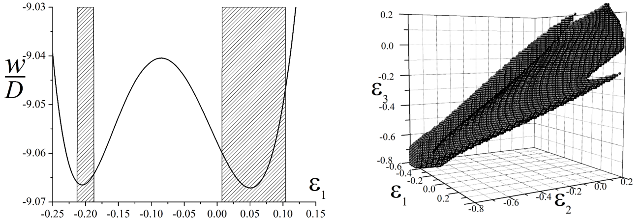
Рис. 4: Слева : Профиль потенциальной энергии деформации, на прямой, соединяющей недеформированную ОЦК (левый минимум) и деформированную ГЦК (правый минимум) решетки; сечение области устойчивости заштриховано. Справа : область устойчивости ГЦК решетки, сглаженный потенциал Морзе \theta = 4.2 , a_{cut} = 5a .
