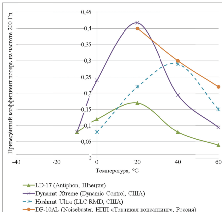
Рисунок 1. Зависимость коэффициента потерь вибропоглощающих покрытий от температуры
