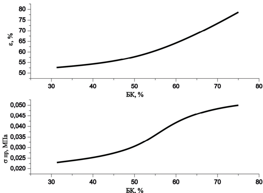
Рисунок 4. Зависимость предела прочности \sigma_{пр} и относительной деформации \varepsilon от содержания БК в матрице композита
