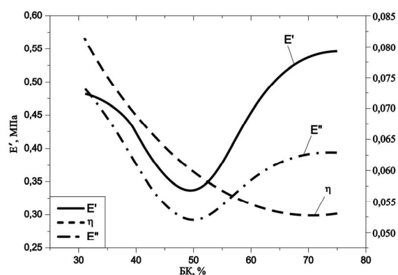
Рисунок 2. Зависимость модуля накопления E' , модуля потерь E'' и коэффициента потерь \eta от содержания БК в матрице композита
