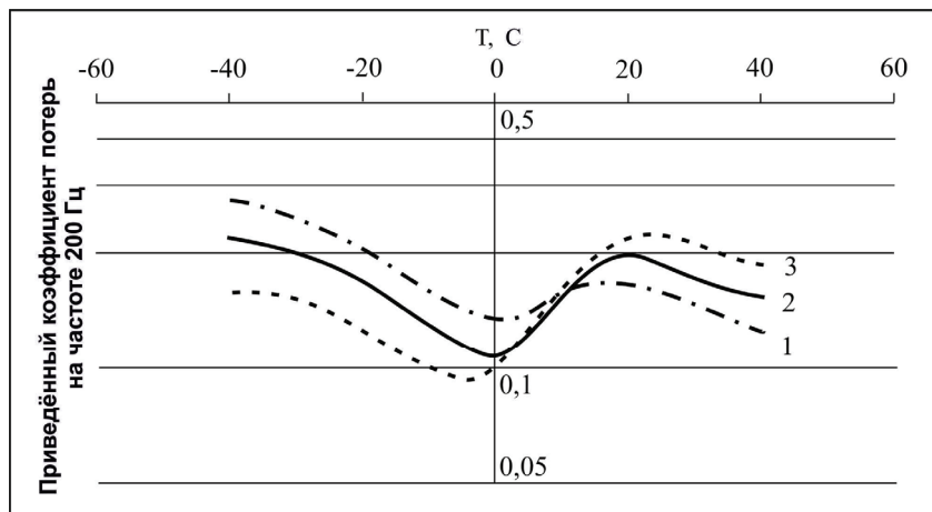
Рисунок 5. Температурная зависимость коэффициента потерь \eta от соотношения в смеси битум:БК (мас. ч.): 1 – 1:3; 2 – 1:1; 3 – 3:1
