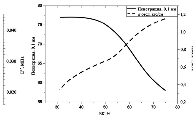
Рисунок 3. Зависимость пенетрации и напряжения при отслаивании от содержания БК в матрице композита
