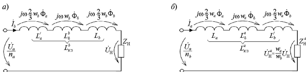
Рис. 4. Упрощенная схема замещения повышающего автотрансформатора относительно тока \dot{I}_b (а) и тока \dot{I}_a (б)
