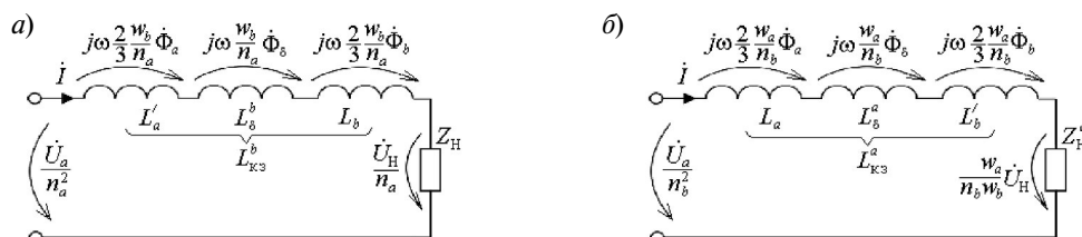
Рис. 5. Упрощенная схема замещения повышающего автотрансформатора относительно тока \dot{I} с индуктивностью КЗ L_{кз}^b (а) и индуктивностью КЗ L_{кз}^a (б)
