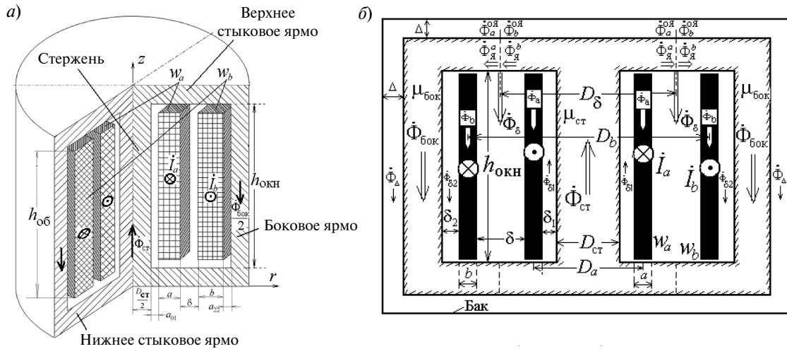
Рис. 2. Магнитная система (а) и расположение обмоток в броневом автотрансформаторе с цилиндрическим боковым яром (б)
