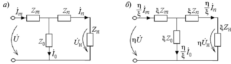
Рис. 6. Преобразование схемы (а) в родственную эквивалентную схему (б)
