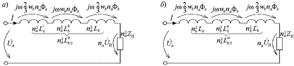
Рис. 7. Упрощенная схема замещения повышающего автотрансформатора относительно входных величин тока \dot{I}, \dot{U}_a с индуктивностью КЗ n_a^2 L_{кз}^b (а) и ее дубликат с индуктивностью КЗ n_b^2 L_{кз}^a (б)
