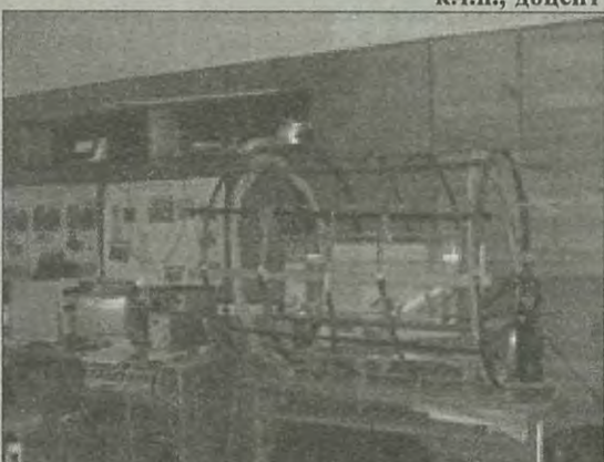
Установка для изучения воздействия переменного магнитного поля на рыб в лаборатории исследований электромагнитных воздействий на природные системы и технические объекты учебного центра «Мониторинг и реабилитация природных систем»
