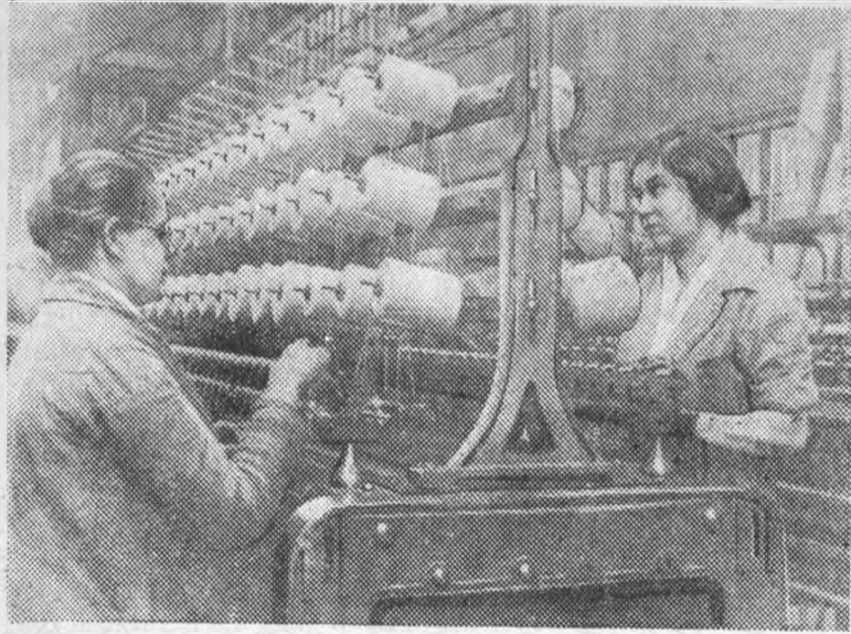
Экспериментальным цехом завода им. Карла Маркса закончен сборкой и установлен на испытание хлопчатобумажный крутильный ватер новой конструкции марки «ВК-66 С».
