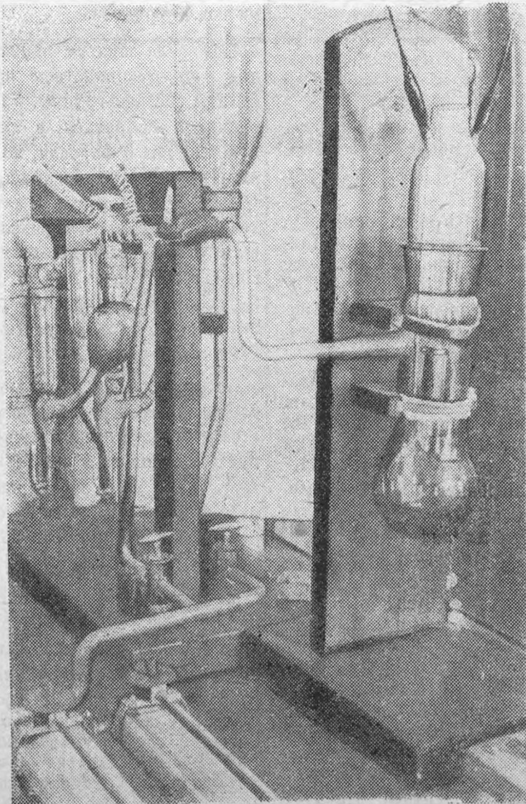
В лаборатории инженерно-физического факультета. На снимке: прибор для нанесения металлов испарением в вакууме (демонстрировался на совещании созданном кафедрой „экспериментальная физика“.
