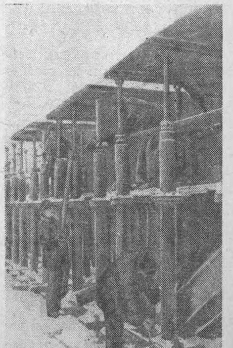
На шахте им. Сталина (Прокопьевск, Новосибирская область) заканчивается монтаж передвижного металлического крепления для работы в лавах, сконструированного по инициативе управляющего шахтой тов. М. Делова и помощника главного инженера тов. С. Милья. На снимке: монтаж металлического крепления
