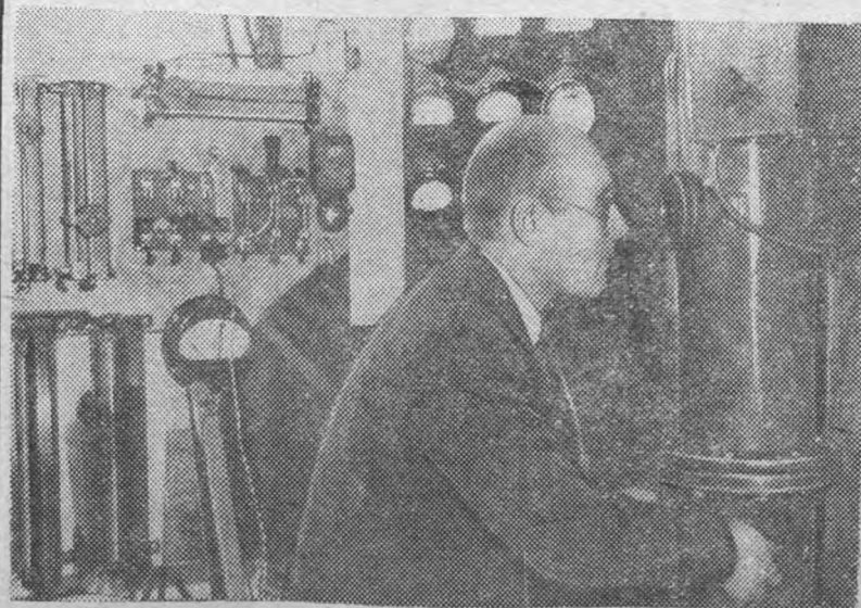
Старший инженер бюро Куйбышевских работ тов. И. Е. Бальгин налаживает катодный осциллограф для записи сверхвысоких напряжений в высоковольтной лаборатории
