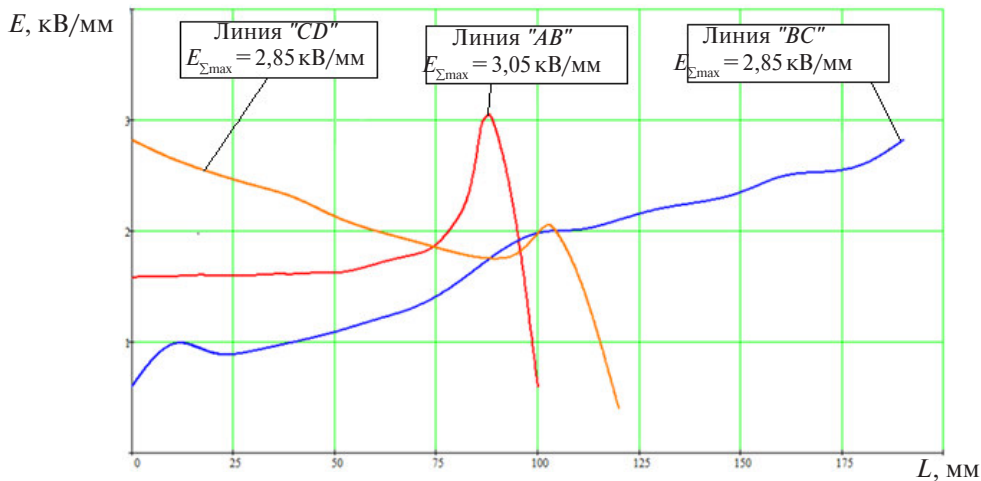
Рис. 8. Распределение модуля напряжённости электрического поля вдоль расчётных контуров усиливающей изоляции
