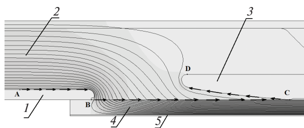
Рис. 7. Диаграмма распределения модуля напряжённости электрического поля
