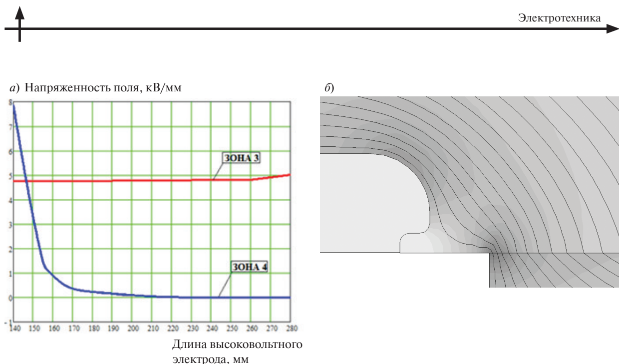
Рис. 2. Зависимости напряженностей электрического поля от длины высоковольтного электрода в зонах 3 и 4 (а) и цветовая диаграмма распределение напряженности электрического поля у края высоковольтного электрода (зона 3) (б). Длина электрода 140 мм
