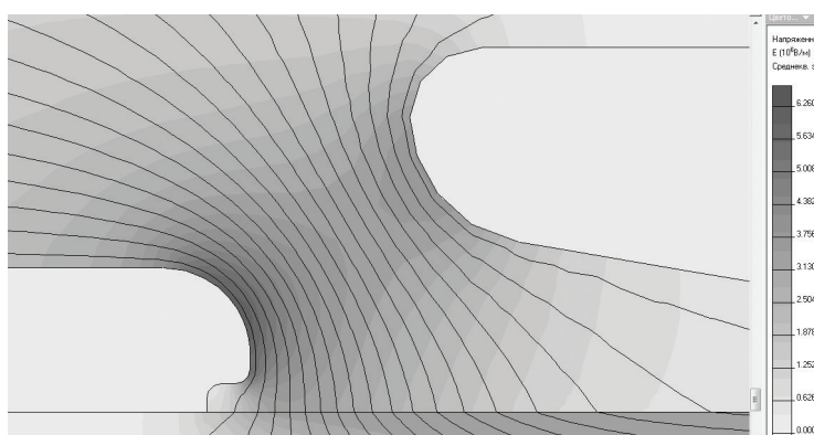
Рис. 5. Распределение напряженности электрического поля между диффлектором и высоковольтным электродом
