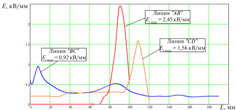
Рис. 9. Распределение тангенциальной составляющей напряжённости электрического поля вдоль расчётных контуров усиливающей изоляции
