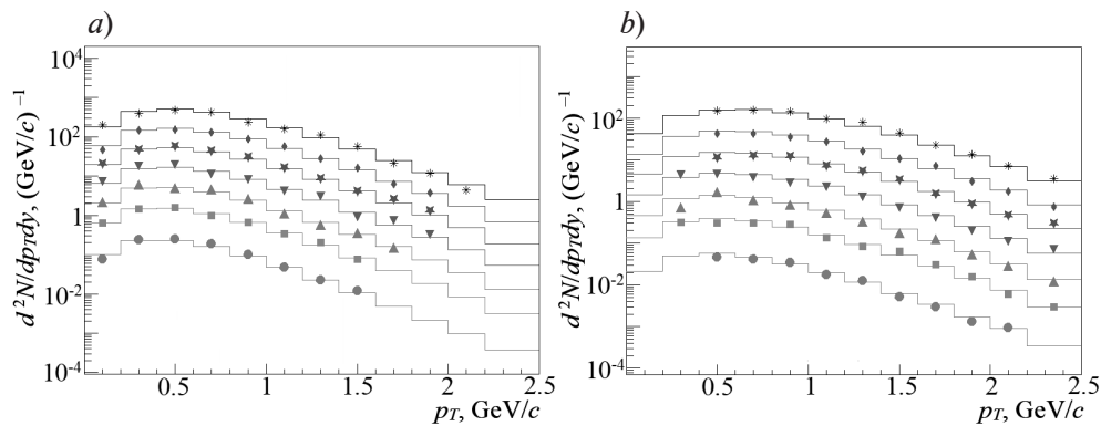
Рис. 5. Восстановленные спектры по поперечному импульсу (символы) и аналогичные спектры, первоначально сгенерированные генератором событий (линии) для K^*(892)^\pm - (a) и \Sigma(1385)^\pm (b) -резонансов в области быстрот |y| < 0,5 .
