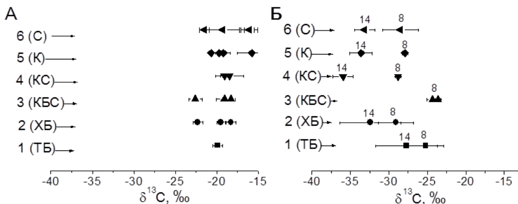
Рисунок 3 – Значения \delta^{13}\text{C} : А – для воздуха около 8-дневного овса, Б – для листьев 8 и 14-дневного овса, освещаемого 1 – теплым белым (ТБ), 2 – холодным белым (ХБ), 3 – красно-бело-синим (КБС), 4 – красно-синим (КС), 5 – красным (К), 6 – синим светом (С)
