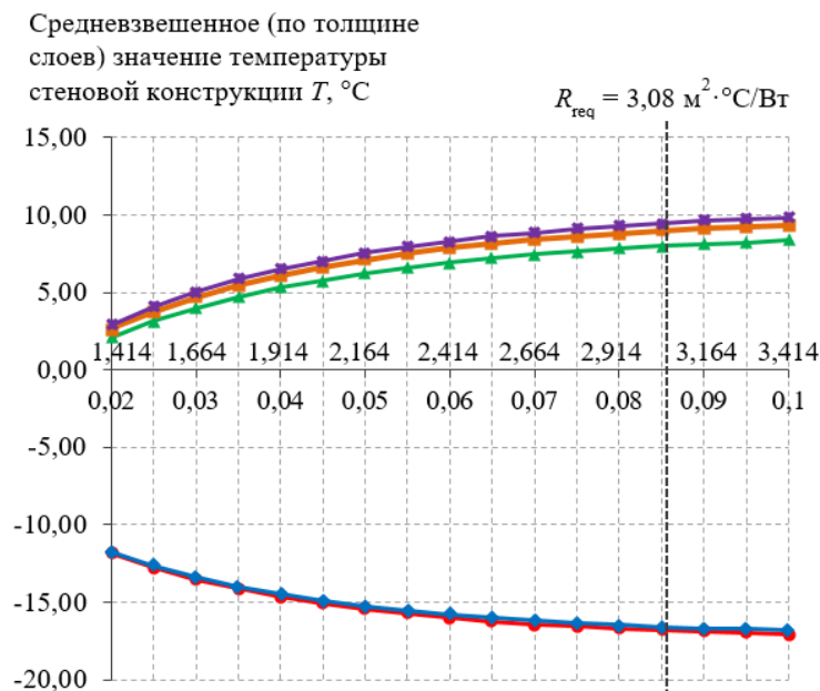
Рисунок 3 – Зависимость теплотехнических характеристик стеновой конструкции от расположения и толщины слоя теплоизоляционного материала
