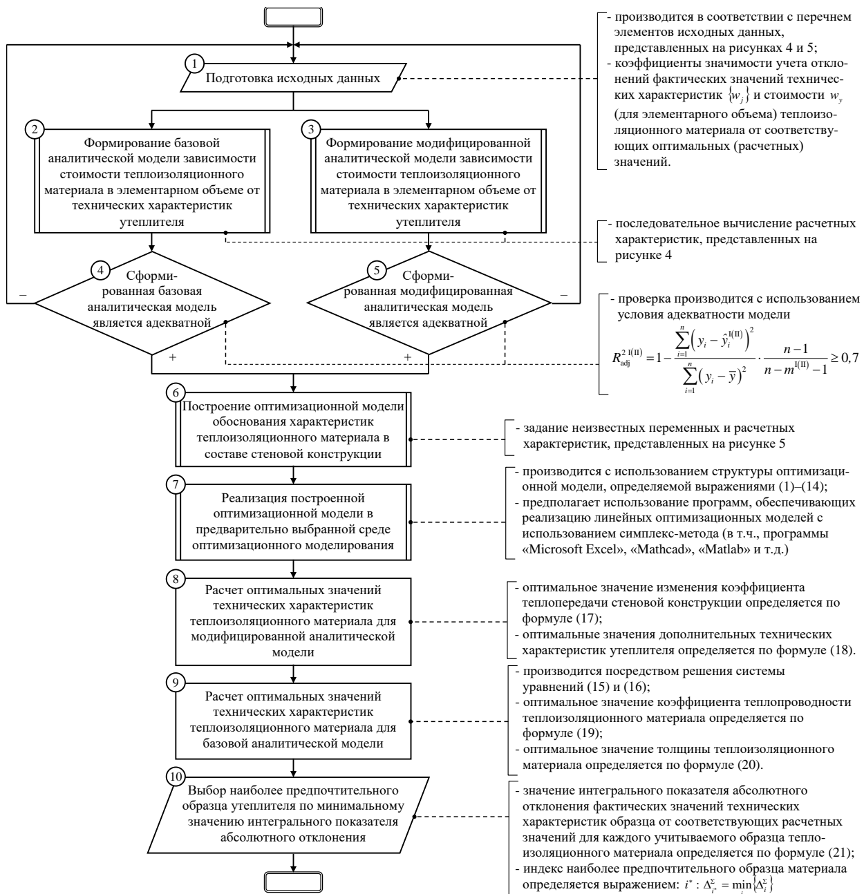
Рисунок 6 – Блок-схема методики обоснования теплотехнических характеристик стеновых конструкций жилых зданий
