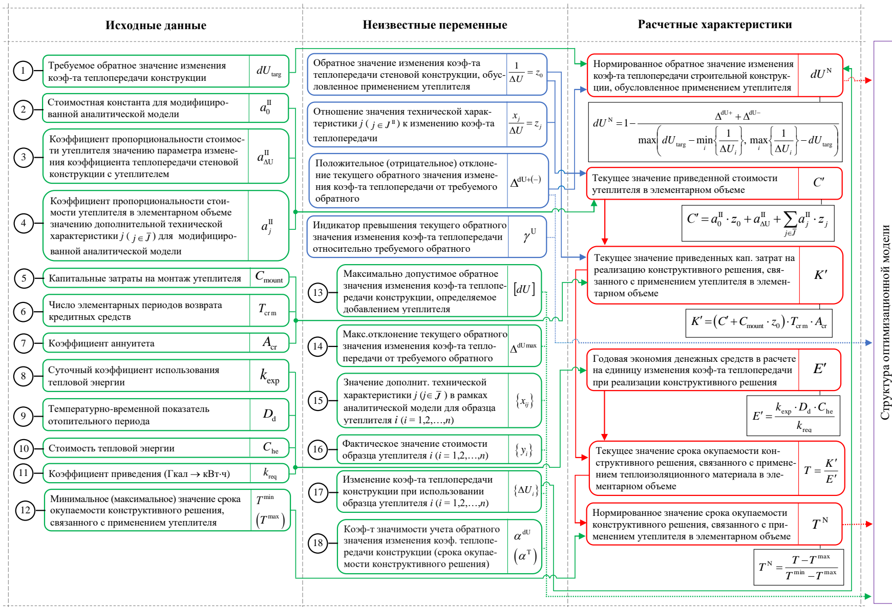
Рисунок 5 – Исходные данные, неизвестные переменные и расчетные характеристики оптимизационной модели
