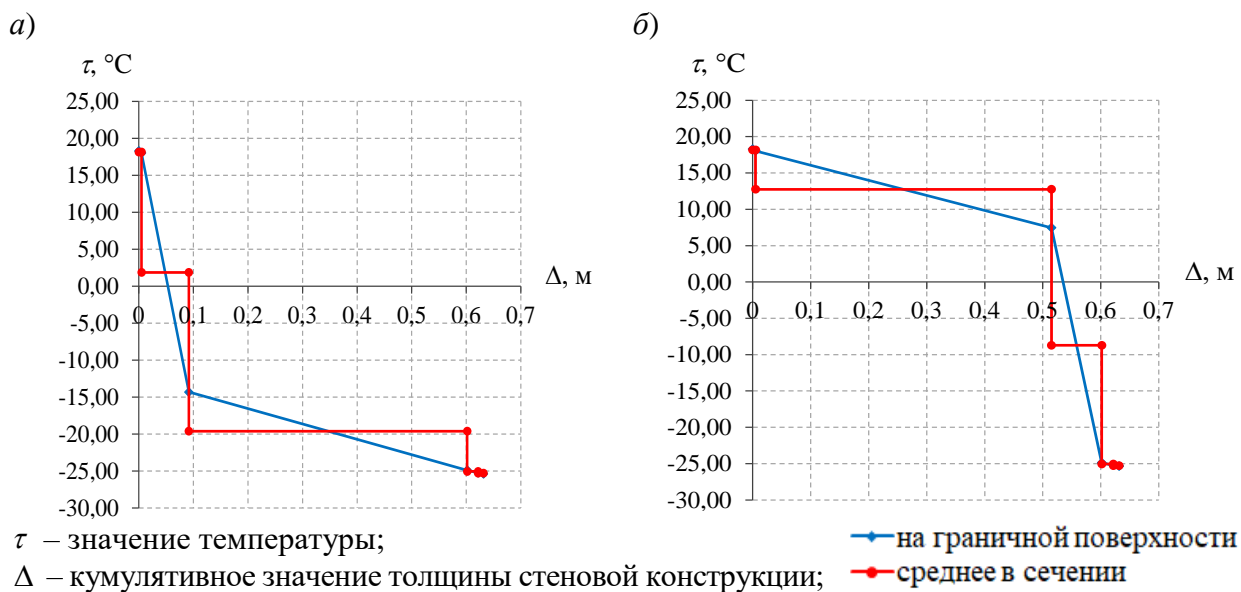
Рисунок 2 – Графики зависимости средней температуры в сечении стеновой конструкции от кумулятивного показателя ее толщины при расположении слоя теплоизоляционного материала: а) – между внутренним (гипсовая штукатурка) и несущим (керамический полнотелый кирпич) слоями; б) – между несущим (керамический полнотелый кирпич) и соединительным (цементно-песчаный раствор) слоями.
