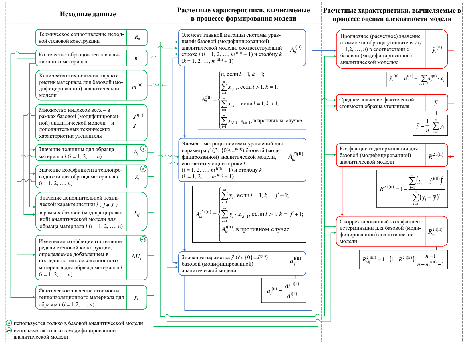
Рисунок 4 – Аналитические модели зависимости стоимости утеплителя от его технических характеристик
