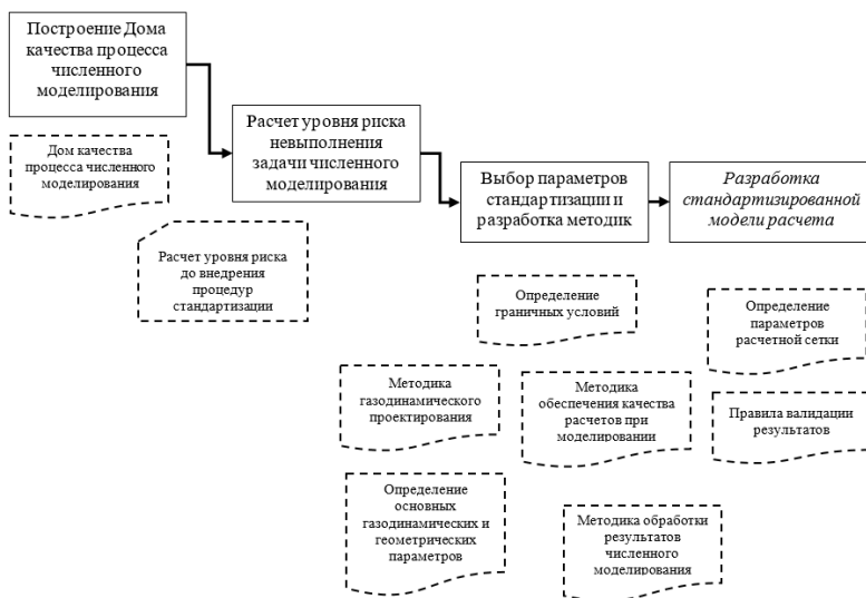
Рисунок 2 – Модель стандартизации процесса численного моделирования малорасходных ступеней центробежных компрессоров
