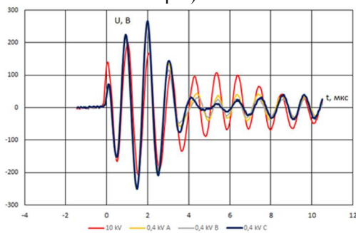
Рисунок 11 – Напряжение обмоток трансформатора 10/0,4 кВ при воздействии колебательного затухающего импульса 1,0 МГц
