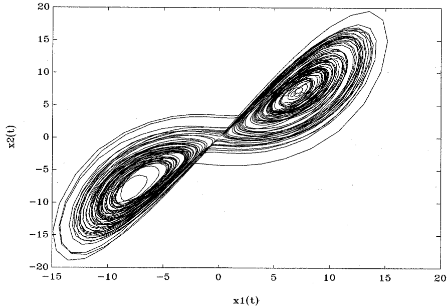
Рис.14.13. Фазовый портрет системы уравнений Лоренца со стохастическим возмущением при b = 8/3 , a = 10 , r = 20.0 , c = 4.0 .
