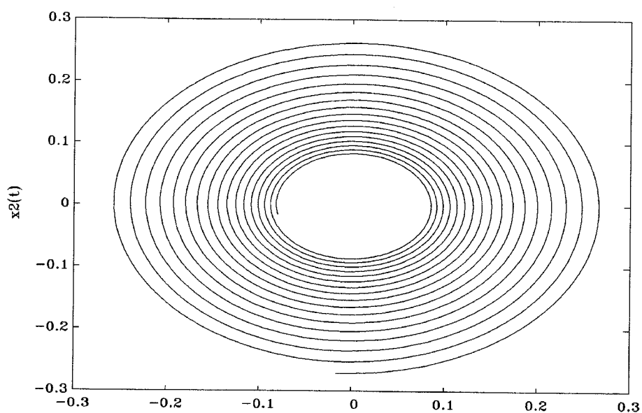
Рис.13.5. Чандлеровские колебания. Фазовый портрет при \lambda = 0.06 , a = 0.0 , \omega = 5.274 .
