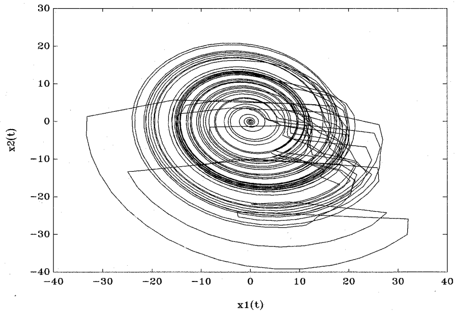
Рис.14.36. Фазовый портрет системы уравнений Рёсслера со стохастическим возмущением при c = 3.77 , e = 0.19 , f = 0.4 , \mu = 8.5 .
