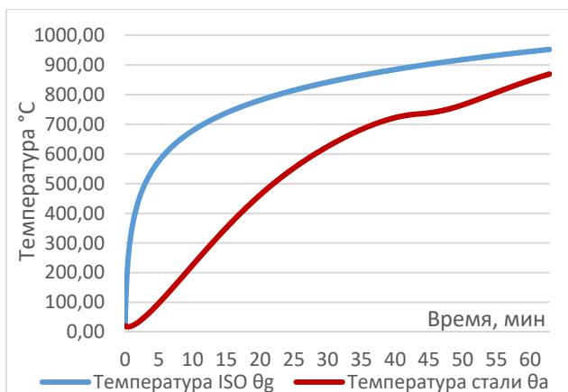
Рисунок 3.18. График роста температуры огнезащищенной конструкции
