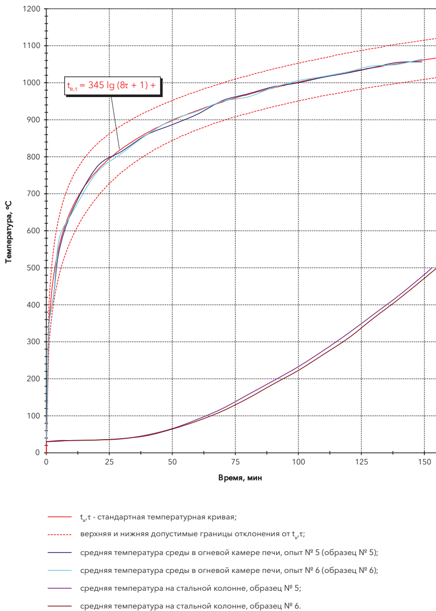
Рис. 4. Температурные кривые прогрева опытных образцов стальных колонн (двутавр № 20) с композицией огнезащитной выполненной из плит теплоизоляционных из минеральной (каменной) ваты CONLIT SL 150 толщиной 80 мм и клея CONLIT Glue.
