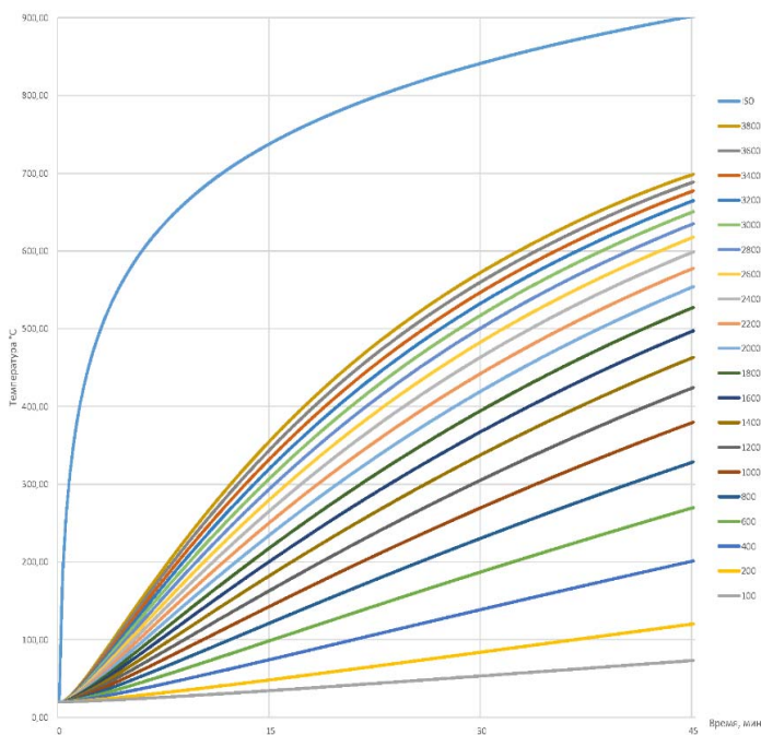
Рисунок 2.12. Модифицированный фрагмент номограммы 2.9 для предела огнестойкости 45 мин для профилей с термическим коэффициентом до 3000.
