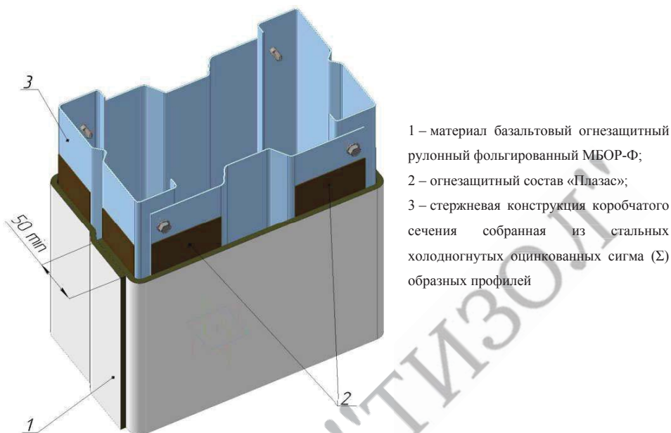
Рисунок 2. Схема огнезащиты конструкции замкнутого профиля
