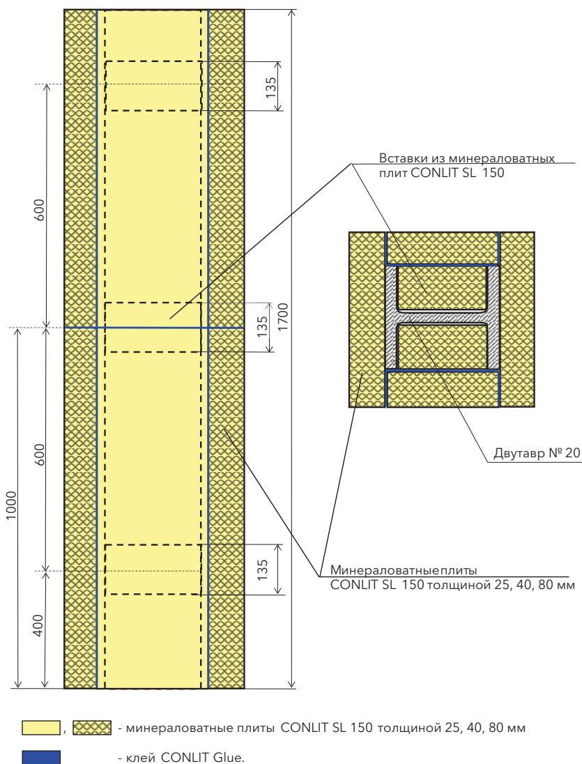
Рис. 1. Схема монтажа однослойной облицовки из минеральной (каменной) ваты CONLIT SL 150 толщиной 25, 40, 80 мм в композиции с клеем CONLIT Glue на опытных образцах стальных колонн
