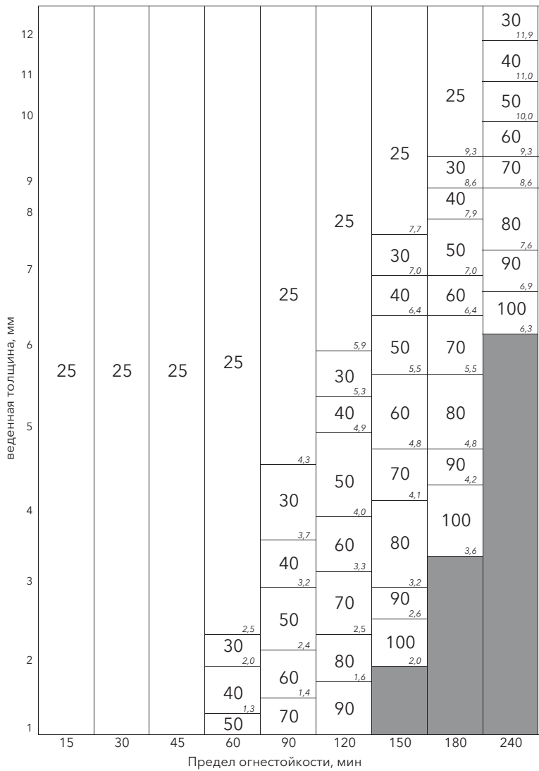
Рис. 10. Толщина материала CONLIT SL 150 в зависимости от предела огнестойкости и приведенной толщины металла
