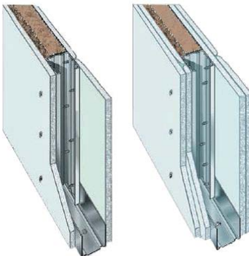
Рисунок 2.2. Решение огнезащиты перегородок ООО «Кнауф ГИПС»
