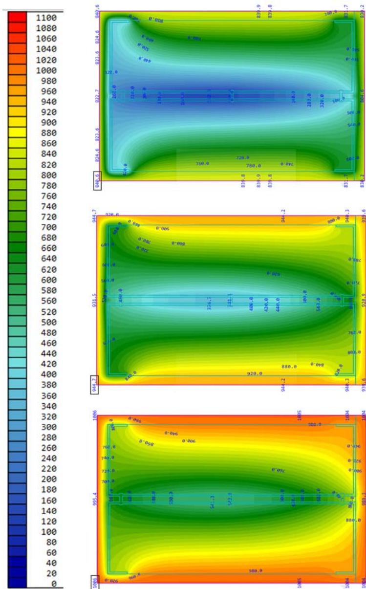
Рисунок 3.12. Градиент температуры на 30, 60 и 90 минуте
