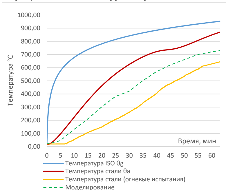
Рисунок 3.23. Кривые огневого воздействия (расчетные и фактические)
