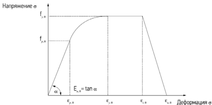
Рисунок 1.6. Диаграмма деформирования углеродистых сталей при повышенных температурах
