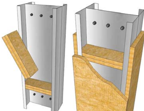
Рисунок 2.4. Решение огнезащиты колонн ООО «ROCKWOOL»
