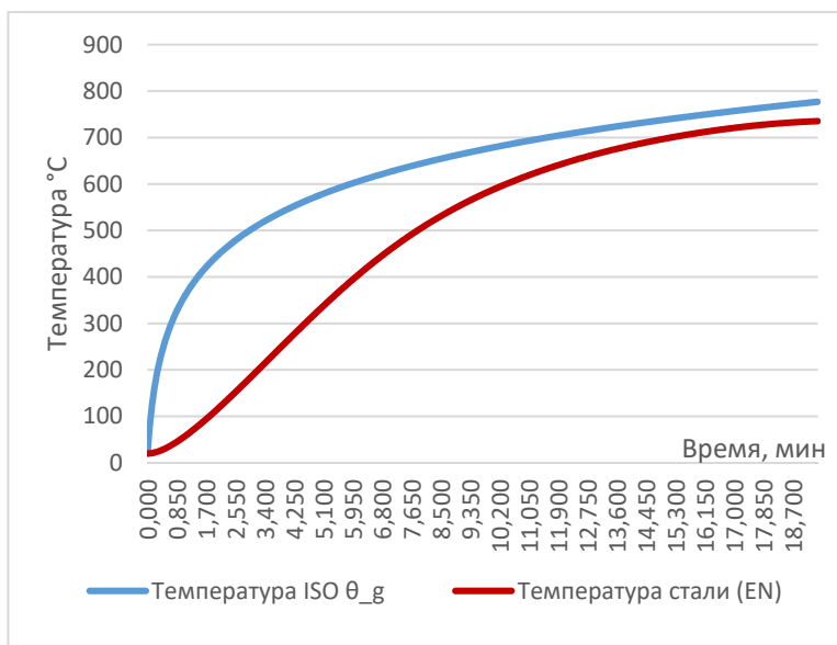
Рисунок 3.2. График роста температуры конструкции
