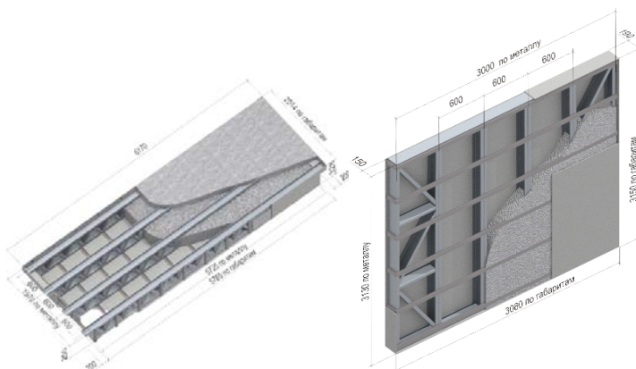
Рисунок 2.5. Решение огнезащиты стен и перекрытий ООО «Андромета»
