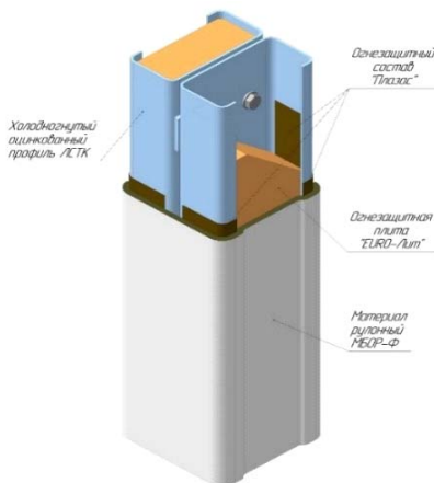
Рисунок 3.8. Решение огнезащиты колонн АО «ТИЗОЛ»
