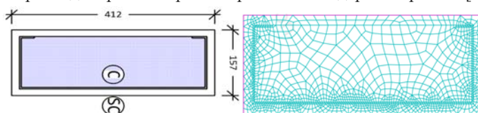
Рисунок 2.13. Расчетная схема конструкции
