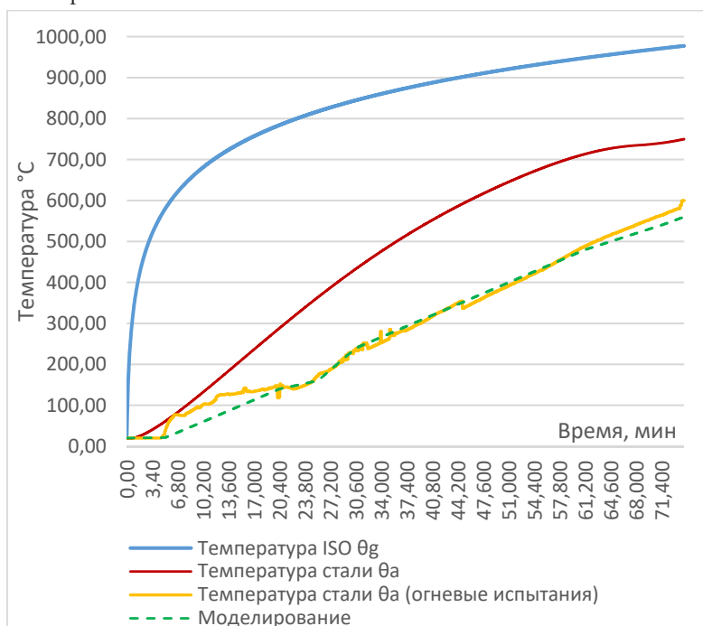
Рисунок 3.15. Кривые огневого воздействия (расчетные и фактические)
