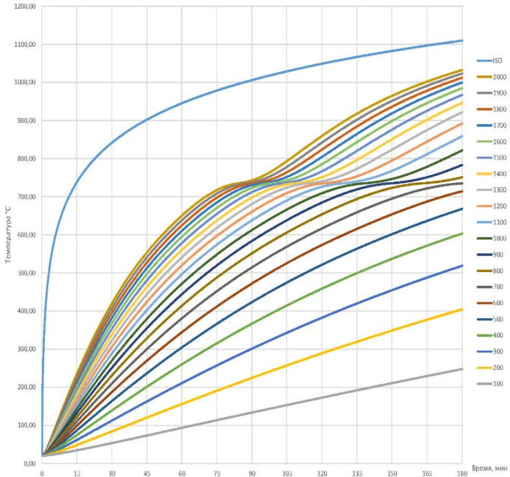
Рисунок 2.9. Номограмма зависимости температуры огнезащищенных стальных конструкций с различными коэффициентами сечения от времени при воздействии стандартного температурного режима
