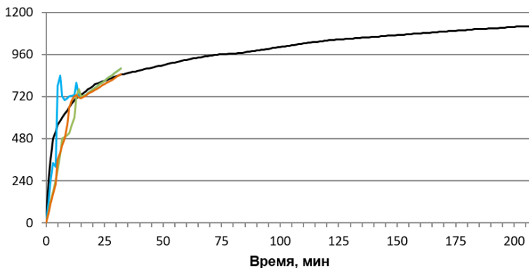
Рисунок 4.3. График изменения температур в огневой камере и показатели термодатчиков на колонне
