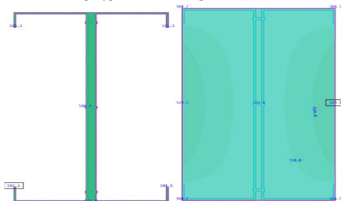
Рисунок 3.4. Градиент температуры для 1-го и 2-го варианта на 8й минуте
