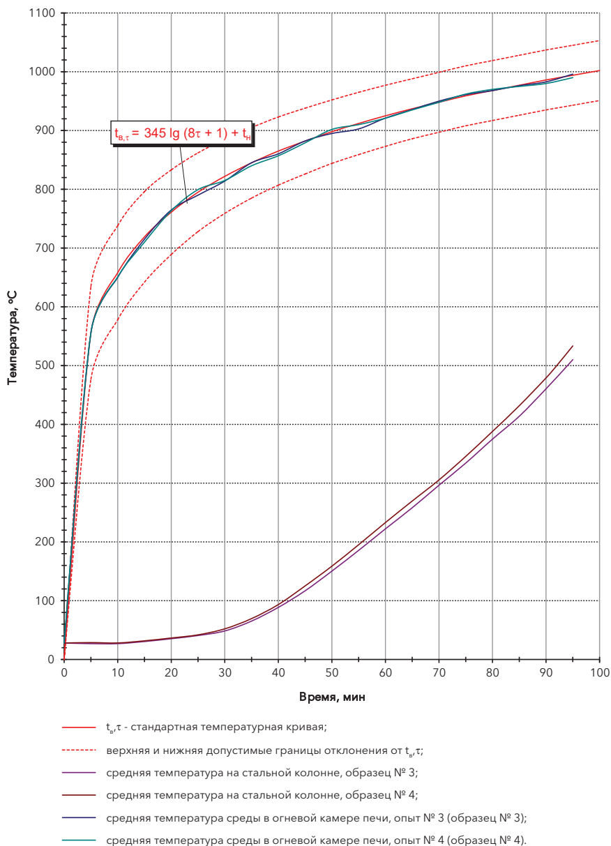
Рис. 3. Температурные кривые прогрева опытных образцов стальных колонн (двутавр № 20) с композицией огнезащитной выполненной из плит теплоизоляционных из минеральной (каменной) ваты CONLIT SL 150 толщиной 40 мм и клея CONLIT Glue.
