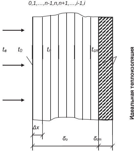
Рис. 9. Схема к расчету на ЭВМ прогрева стальной пластины с огнезащитной облицовкой.
