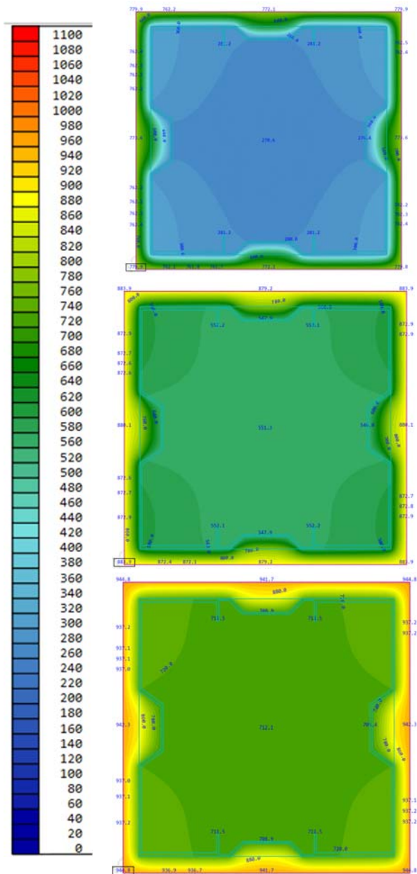
Рисунок 3.20. Градиент температуры на 20, 40 и 60 минуте
