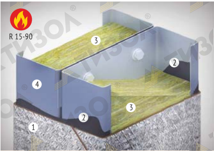
Огнезащита конструкций из профилей, собранных двутавром 1. Материал рулонный МБОР-Ф 2. Огнезащитный состав «ПЛАЗАС» 3. Огнезащитная плита «ЕВРО-ЛИТ» 4. Холодногнутый оцинкованный профиль ЛСТК
