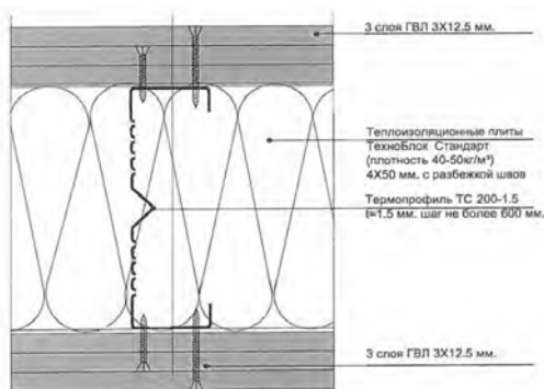
Рисунок 3.25. Моделируемый фрагмент образца стены
