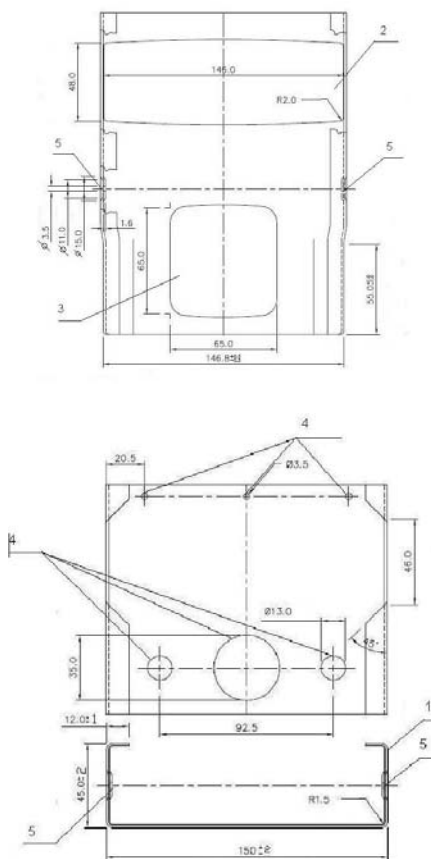
Рис. 4. Схема расположения отверстий и вырезов в исходной заготовке С-образного сечения 1-профиль; 2-отверстие 48х146 мм; 3-отверстие 65х65; 4-круглые отверстия; 5-“пуклевки”
