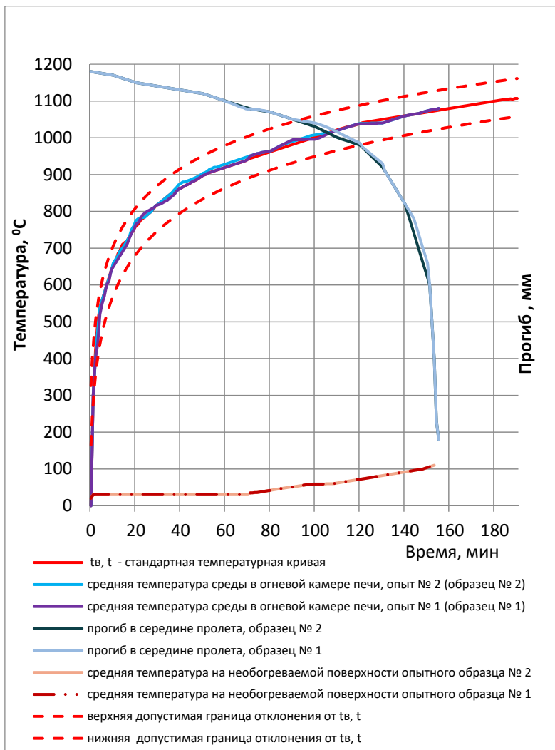
Рис. 3.29 – Графики изменения температур в огневой камере и показатели термомпар на стеновой панели
