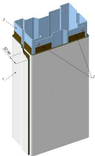
Рисунок 3.17. Решение огнезащиты колонн АО «ТИЗОЛ»
