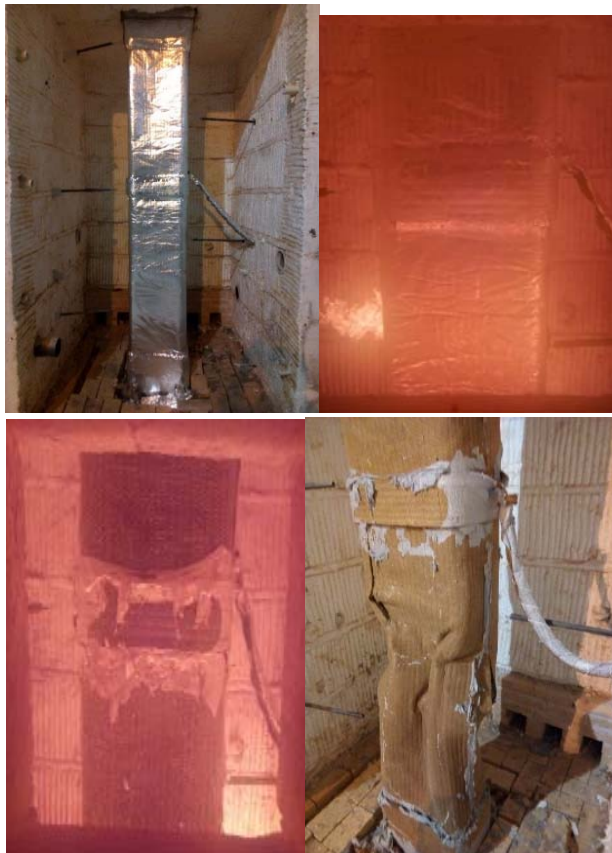
Рисунок 3.13. Испытываемый образец до и после огневого воздействия
