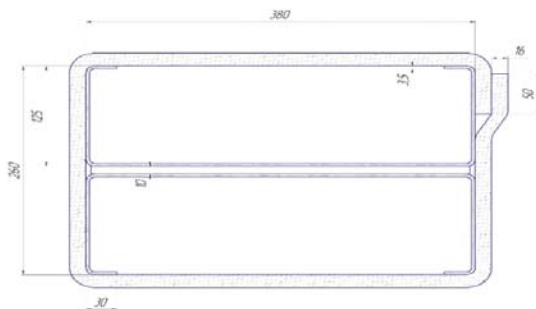
Рисунок 3.9. Расчётная схема составного сечения с огнезащитой
