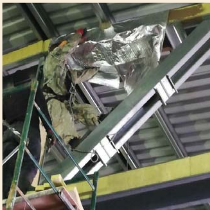
Начало работ по огнезащите ЛСТК
