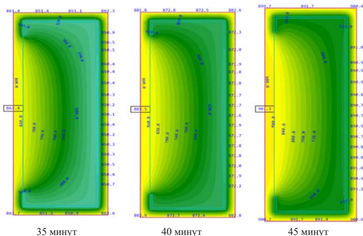
Рисунок 2.14. Моделирование температурного градиента
