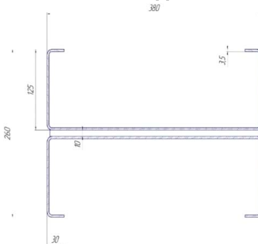
Рисунок 3.1. Схема расчета составного сечения
