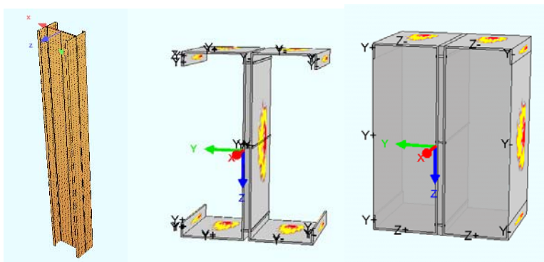
Рисунок 3.3. Смоделированные сечения образца
