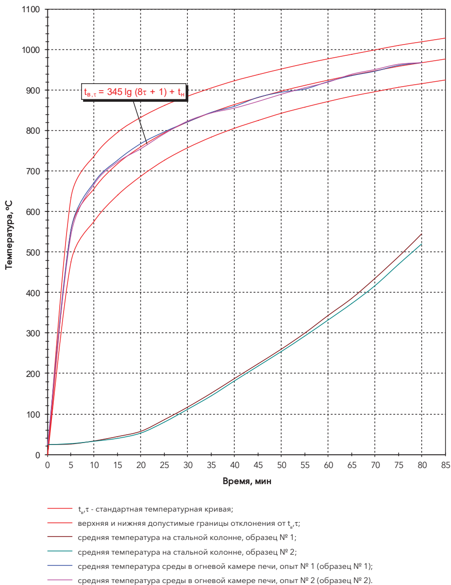
Рис. 2. Температурные кривые прогрева опытных образцов стальных колонн (двутавр № 20) с композицией огнезащитной выполненной из плит теплоизоляционных из минеральной (каменной) ваты CONLIT SL 150 толщиной 25 мм и клея CONLIT Glue.
