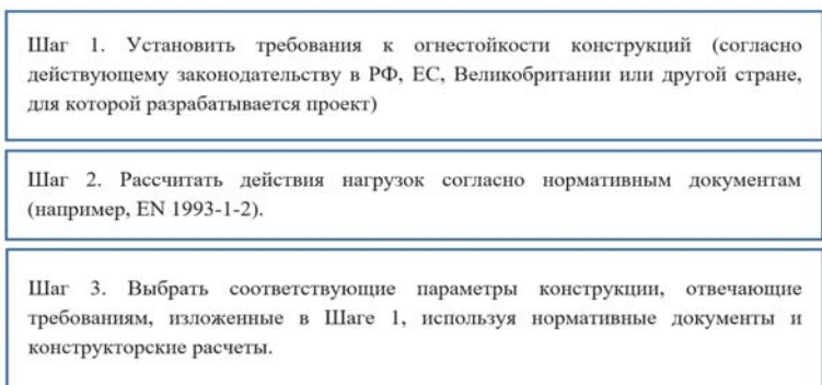
Рисунок 1.2. Упрощенная процедура расчета огнестойкости конструкций
