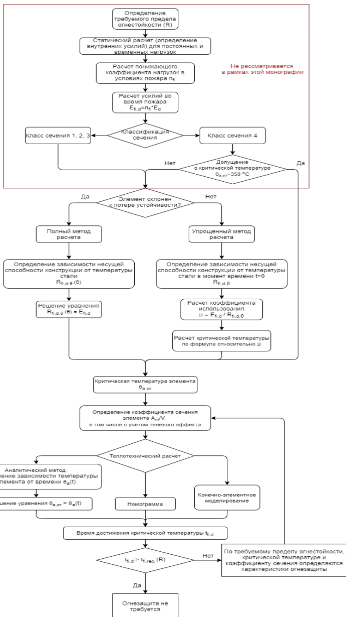
Рисунок 1.4 Алгоритм расчета на огнестойкость и применение огнезащиты
