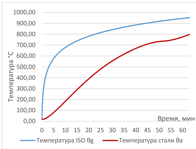
Рисунок 2.11. График прогрева огнезащищённой стальной конструкции
