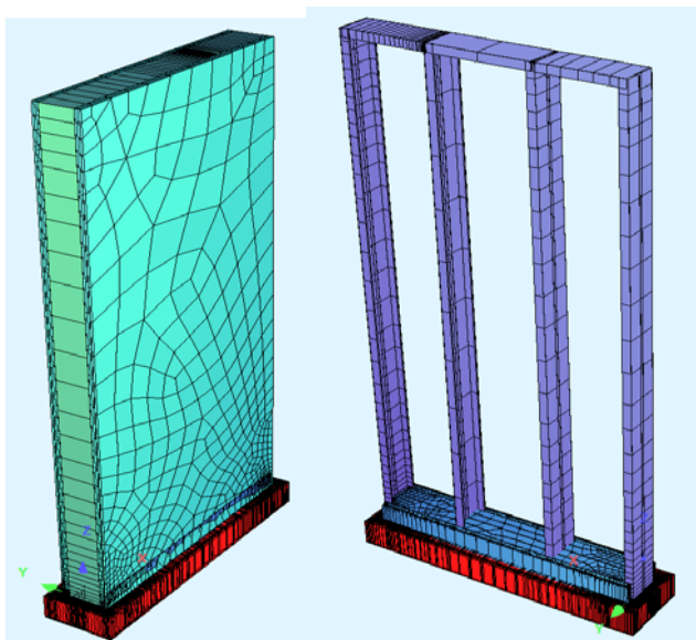
Рис.3.27 Несущая стена на основе ЛСТК-каркаса
