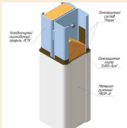
Схема монтажа системы ЕТ ЛСТК
