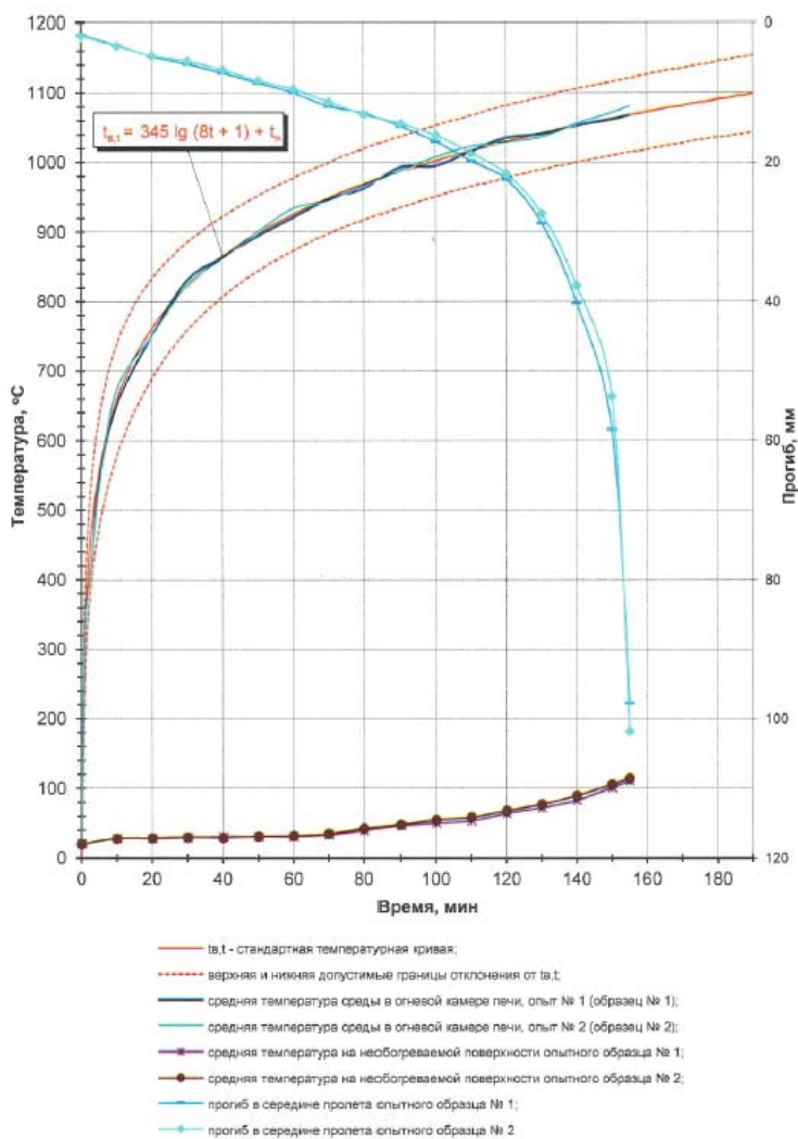
Рисунок 4.9. Графики изменения температур в огневой камере и показатели термодар
