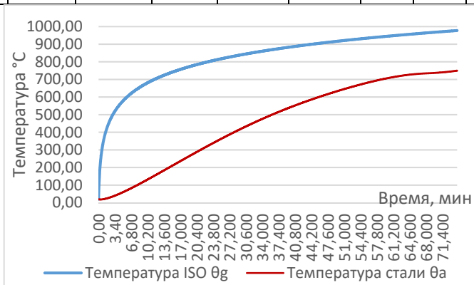
Рисунок 3.10. График роста температуры конструкции с огнезащитой
