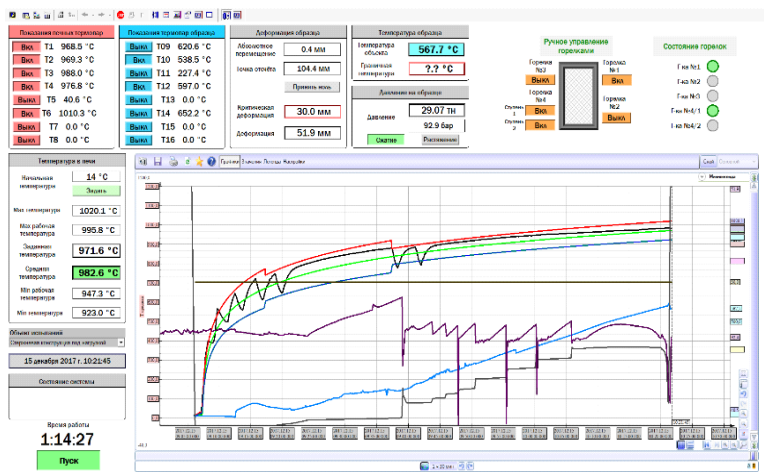
Рисунок 3.14. График изменения значения температур на термопарах. Красная и синяя линия – верхняя и нижняя границы допуска температурного отклонения от кривой ISO; зеленая линия – заданная температура в печи; черная – средняя температура в печи; голубая – средняя температура нагрева образца
