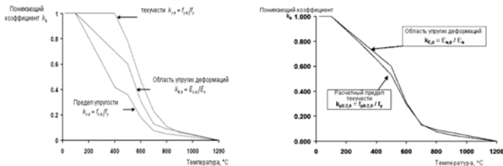
Рисунок 1.7. Изменение коэффициентов снижения для диаграммы деформирования углеродистых сталей при повышенных температурах: а – обычных конструкций, б – для поперечных сечений 4 класса (ЛСТК)
