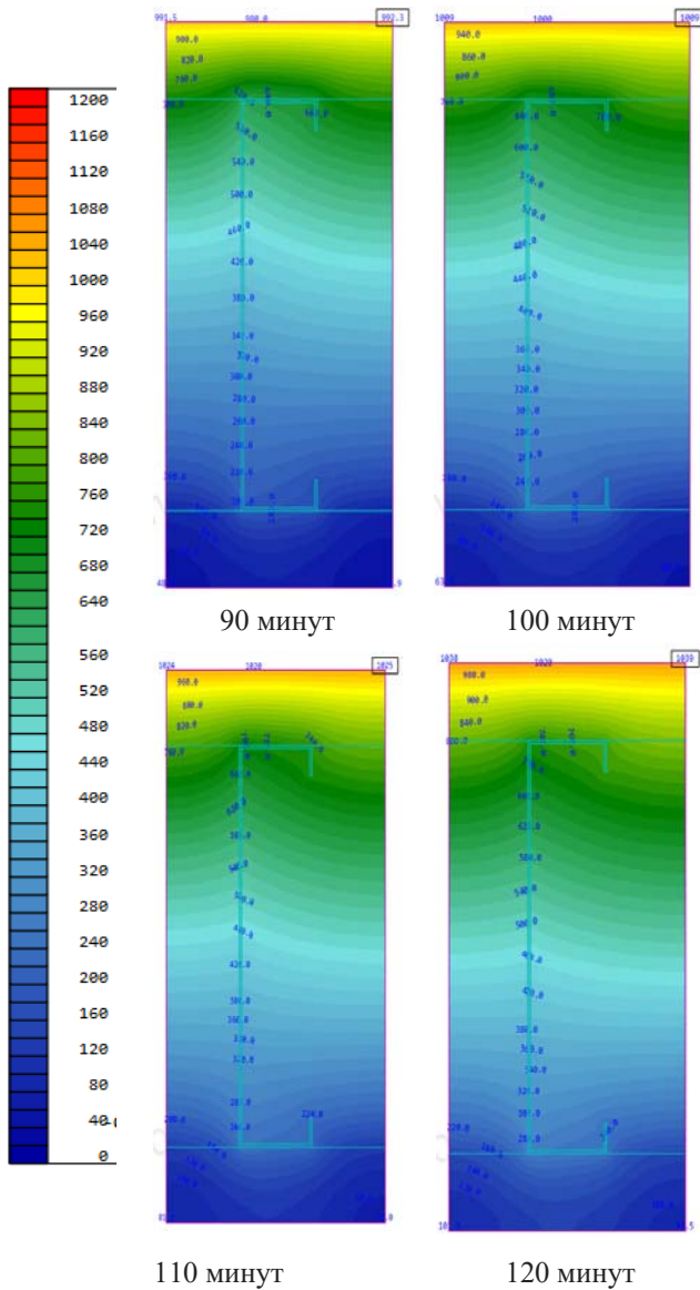
Рис. 3.28. Градиент температур расчетного сечения
