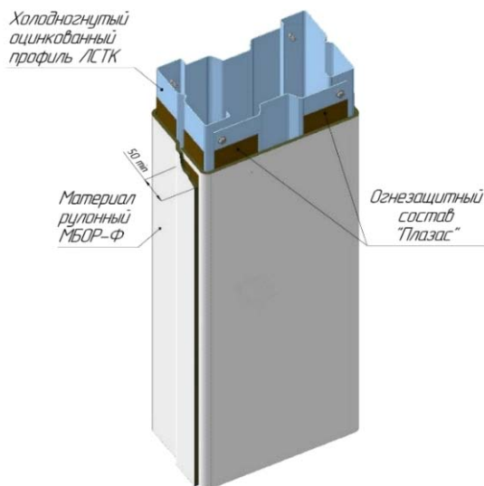
Рисунок 2.3. Решение огнезащиты колонн АО «ТИЗОЛ»
