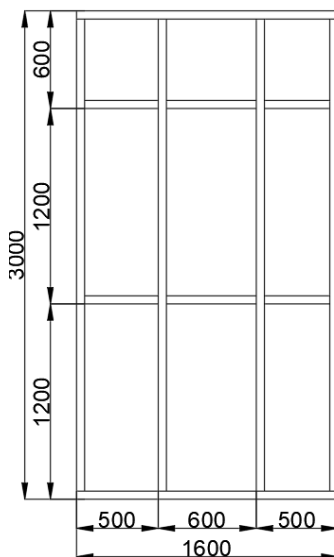
Рисунок 3.24. Схема испытываемого образца стены
