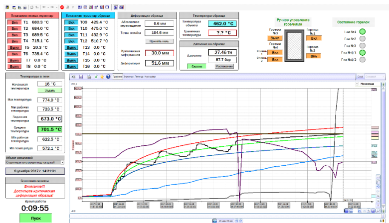
Рисунок 3.6. График изменения значения температур на термонапарх. Красная и синяя линии – верхняя и нижние границы допуска температурного отклонения от кривой ISO; зеленая линия – заданная температура в печи; черная – средняя температура в печи; голубая – средняя температура нагрева образца
