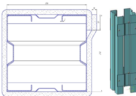
Рисунок 3.16. Расчётная схема составного сечения с огнезащитой
