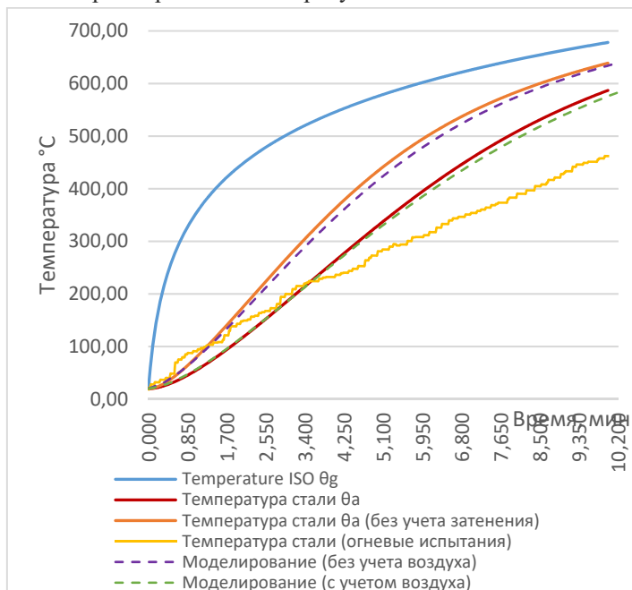
Рисунок 3.7. Кривые огневого воздействия (расчетные и фактические)
