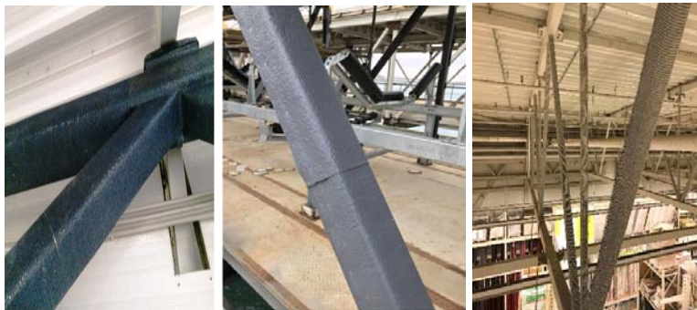
Рисунок 2.6. Защищенные рулонной сеткой стальные конструкции, в том числе и для наружной эксплуатации в морском климате
