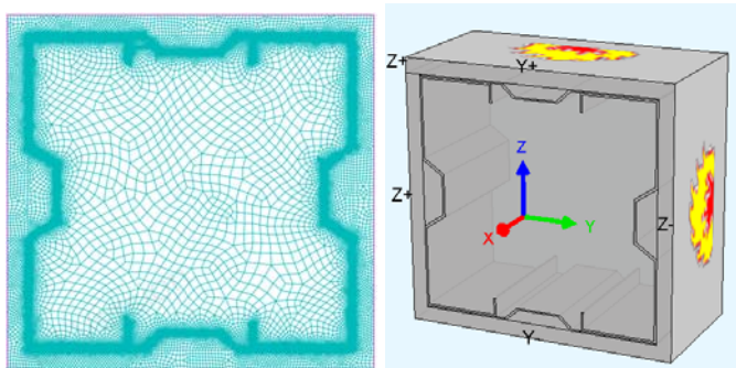
Рисунок 3.19. Смоделированные сечения образца
