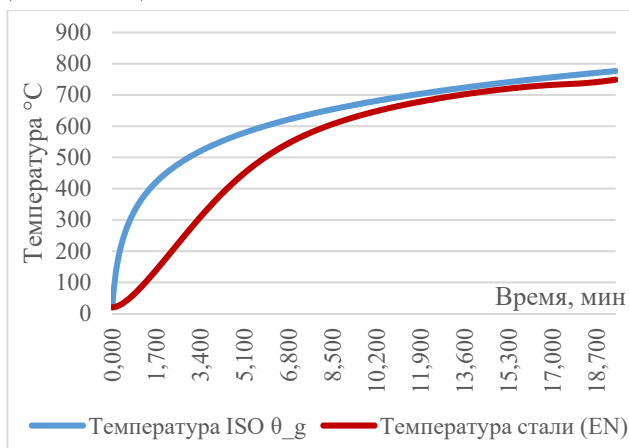
Рисунок 2.8. График прогрева незащищенной стальной конструкции
