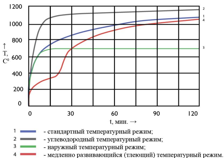
Рисунок 1.5. Кривые, описывающие температурные режимы пожара согласно ГОСТ Р ЕН 1363-2-2014 [26]
