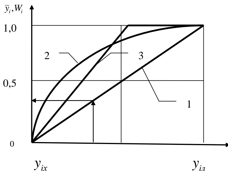
Рис. 18. Функции для построения нормированных значений и оценок критериев нижнего уровня: 1- функция перевода в нормированные значения; 2- предполагаемая оценочная функция; 3- аппроксимация оценочной функции.
