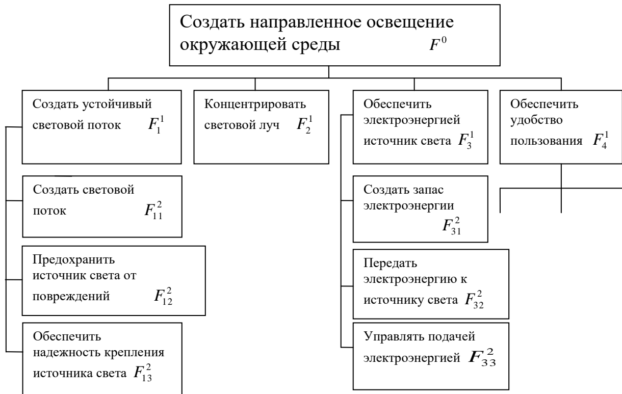
Рис. 3. Дерево функций для ручного фонарика
