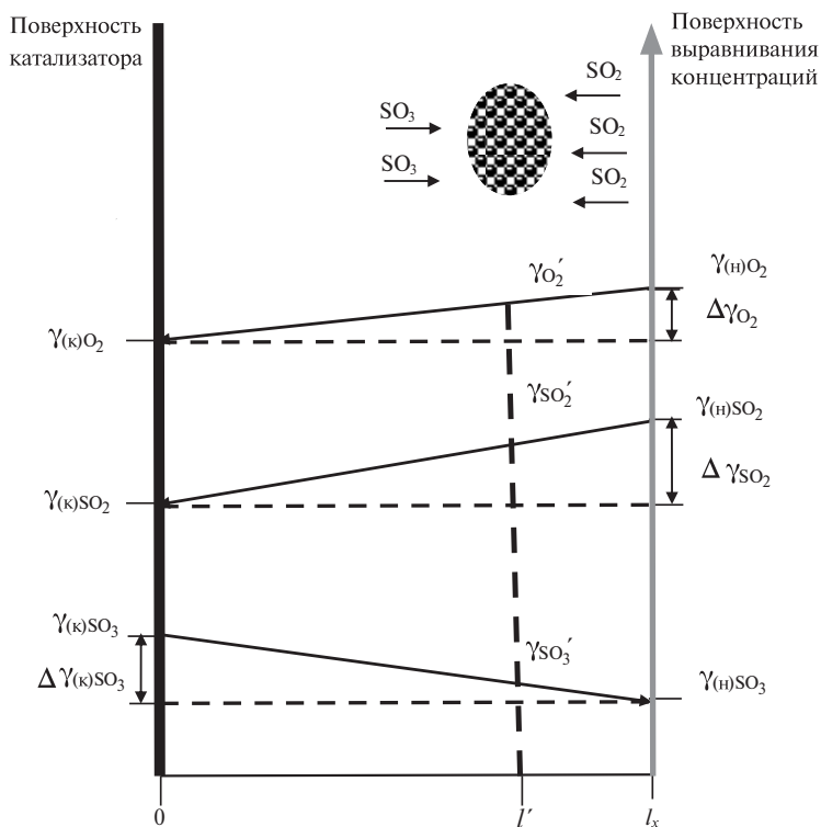
Рис. 1. Перенос аэрозольной частицы к поверхности катализатора, вызванный градиентом концентраций \text{O}_2 , \text{SO}_2 и \text{SO}_3 при реакции окисления:
